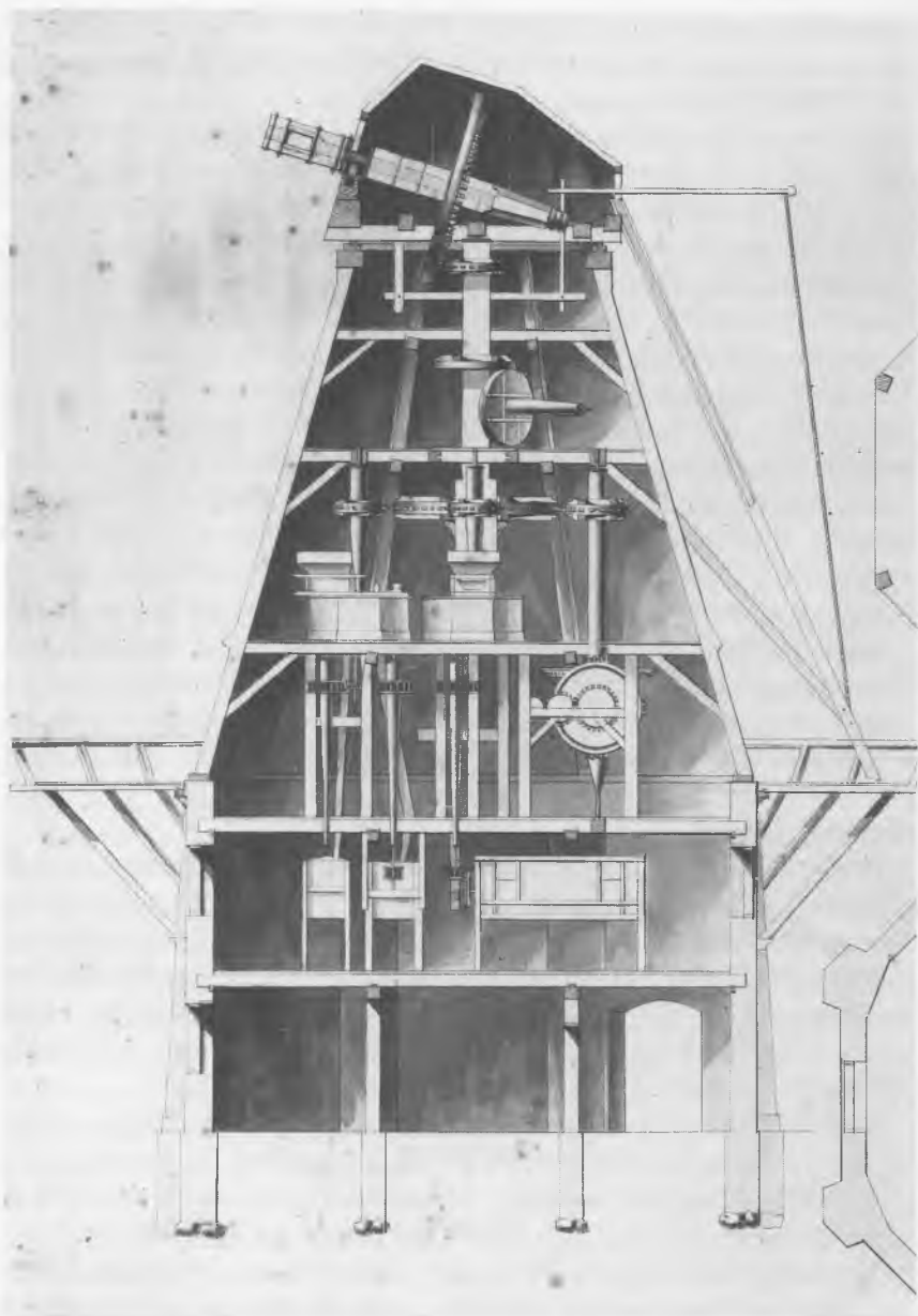
Snit af hollandsk mølle. Tegning ca. 1840 til ukendt mølle af møllebygger Jørgen Jørgensen, København. Nationalmuseet.
