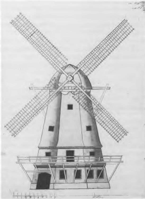
St. Kongens mølle på Schacks bastion. Tegningen fra 1768 er sandsynligvis den ældste bevarede konstruktionstegning til en vindmølle i Danmark. Rigsarkivet.
