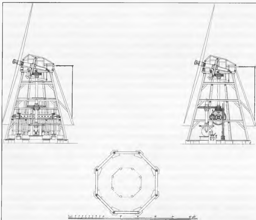
Fredens mølle på Amager. Konstruktionstegning tidligst fra 1805, der viser oliemøllens stampeværk og kollergang til knusning af oliefrø. Kunstakademiet, Samlingen af arkitekturtegninger.
