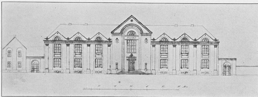
MALLINGS FAÇADETEGNING TIL UNIVERSITETSBYGNINGEN (Stik i Universitetsprogram 1836)
