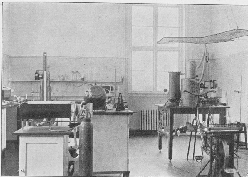
GYMNASTIK-TEORETISK LABORATORIUMS STORE LOKALE FOR ARBEJDSFORSØG
