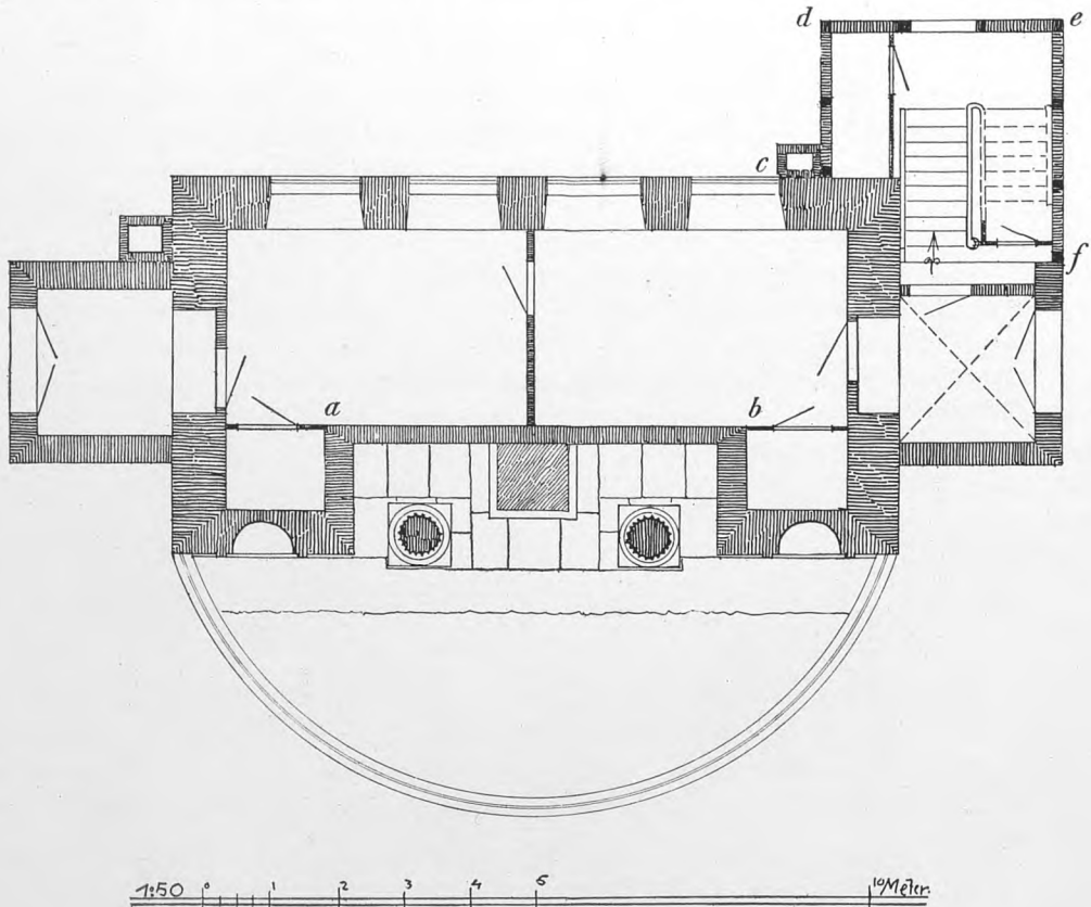
Opmaaling af »Herkuleslogen« i Kongens Have 1913.
