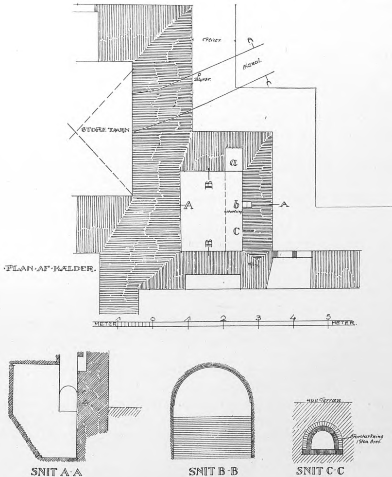
Opmaaling af Kælderen under Christian IV.s W. C. og af Afledningskanal.
