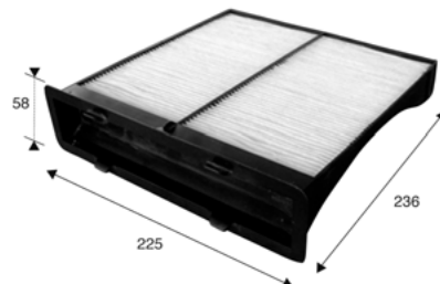
Valeo 715625
