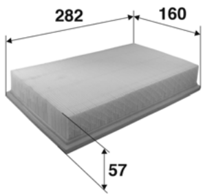
Valeo 585262
