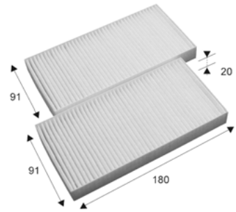
Valeo 715696
