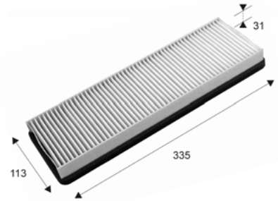
Valeo 715646
