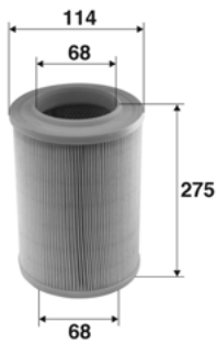
Valeo 585634
