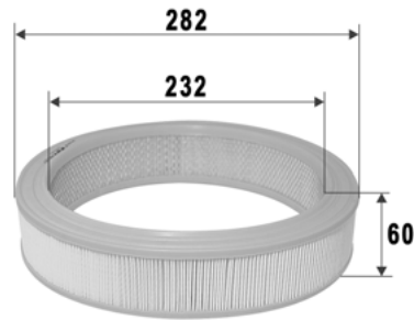
Valeo 585746
