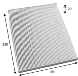
Valeo 715740
