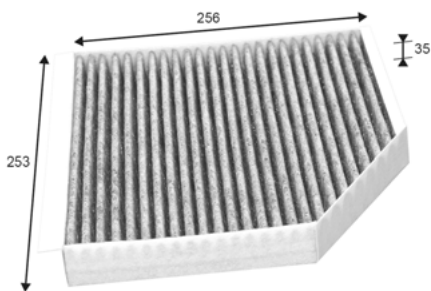
Valeo 715733
