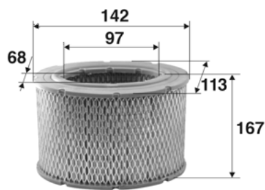
Valeo 585623
