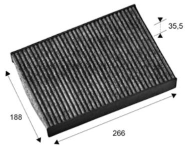
Valeo 701000
