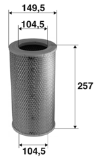
Valeo 585639
