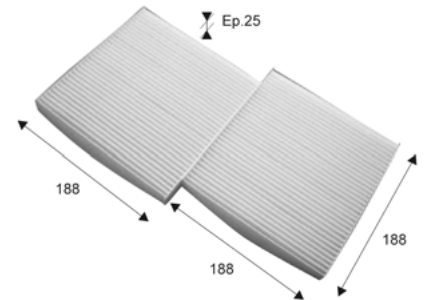
Valeo 715714
