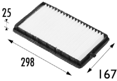
Valeo 698171
