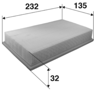
Valeo 585222
