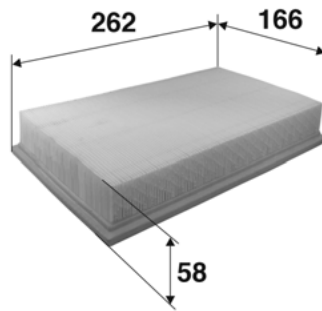
Valeo 585372
