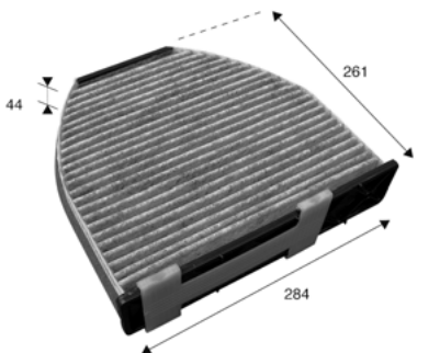
Valeo 715600
