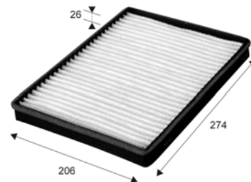
Valeo 715654
