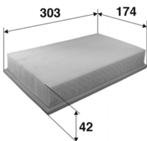
Valeo 585374
