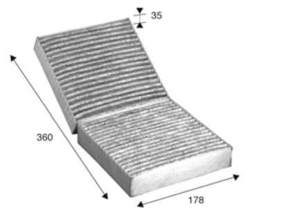
Valeo 715508
