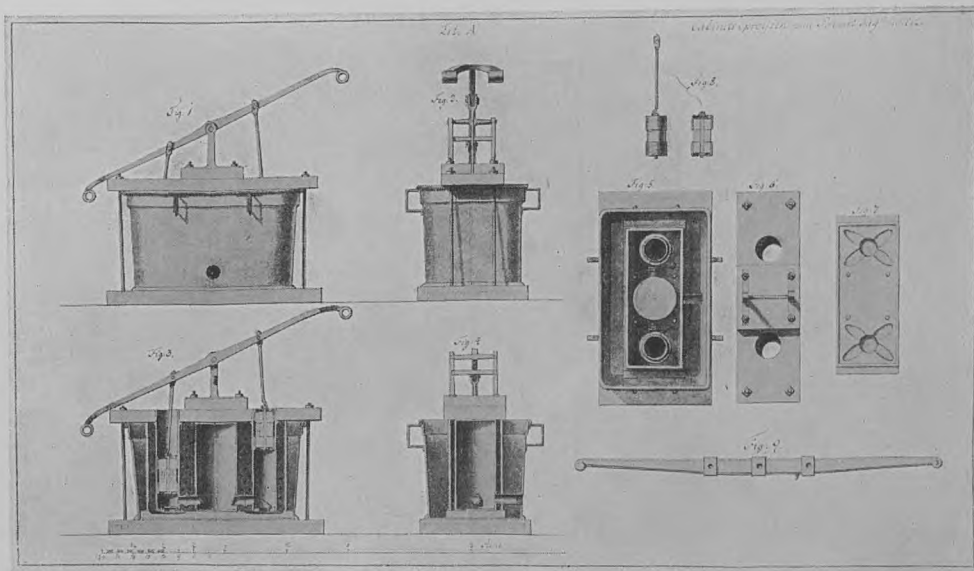
Kabinetssprøjte paa Prinsens Palæ. Tegning. (Hovedbrandstationen).
