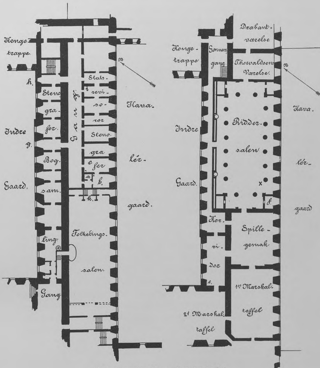
Plan af Mezzanin og Kongens Etage i søndre Fløj.
