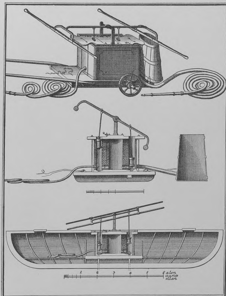
En af de store Sprøjter (foroven) og en Pramsprøjte. Thurah: Hafnia hodierna, 1748, Pl. II.
