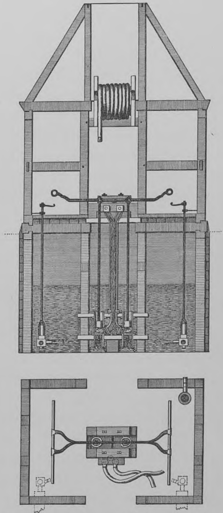
Trykværket ved Nikolaj Kirke. Thurah: Hafnia hodierna, 1748, Pl. III.
