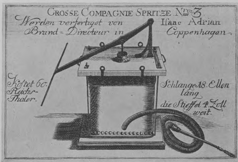
Adrians Sprøjte. (Stik i Raadstuearkivet).
