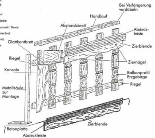
Montagevariante mit Abdeckleiste
