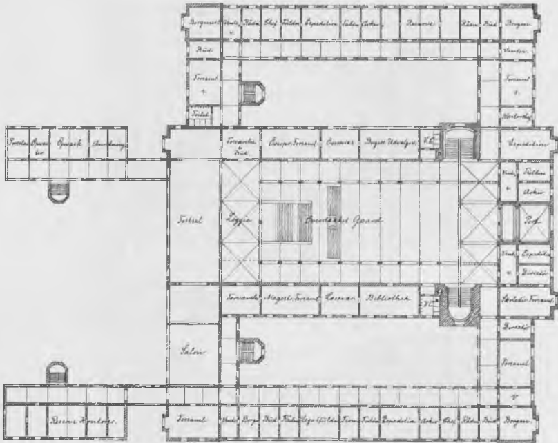
M. Nyrops skitse I B 1891, plan af 1. sal. Facaden mod højre. 1:1200.
