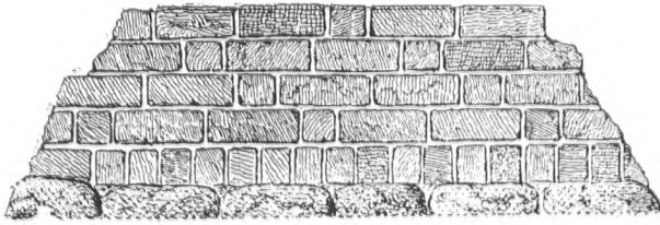
Murstensforbandt fra Valdemarsmuren ved Danevirke.
