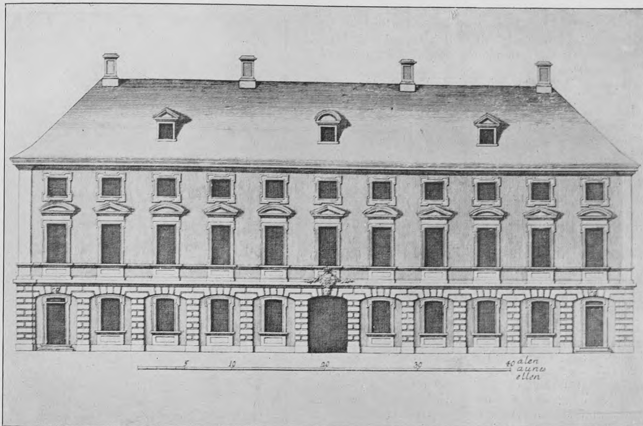
Landetatens Generalkommissariat og Admiralitetet (Størrestræde). Hovedfacade mod Holmens Kanal 1740erne. Se Teksten Side 440. L. Thura: Den danske Vitruvius.
