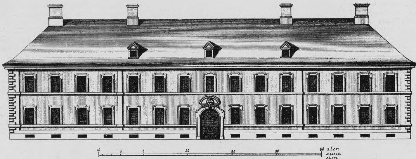
Ældre Opmaaling af Staldmestergaardens Facade mod Frederiksholms Kanal.
