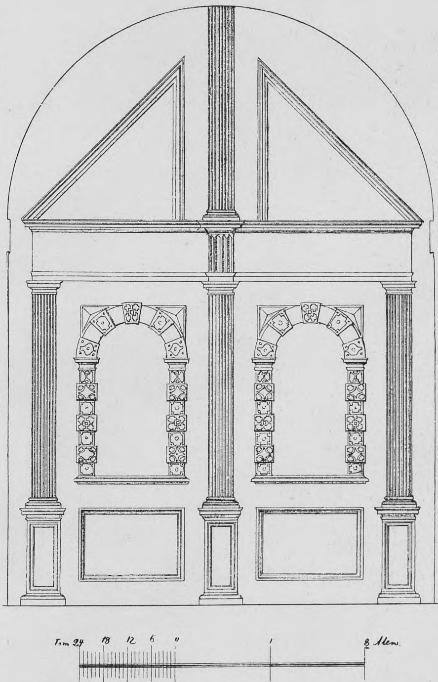
Renaissanceportfløje fra Tøjhusets Port mod Tøjhusgade (opmaalt 1860 af Klein).
