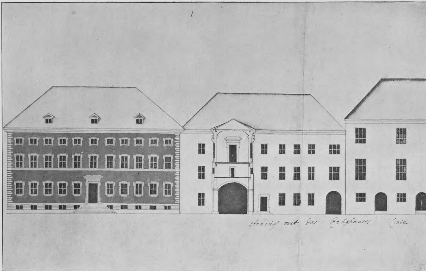
Oprindeligt Forslag til Façader for Kancellibygningen og Fr. IV's Arkivbygning med mellemliggende Proviandhusgavl og Snit gennem Løngangen fra Slottet, og helt til højre Façaden af Fr. III's Biblioteksbygning. Udarbejdet af I. C. Ernst. Rigsarkivet.
