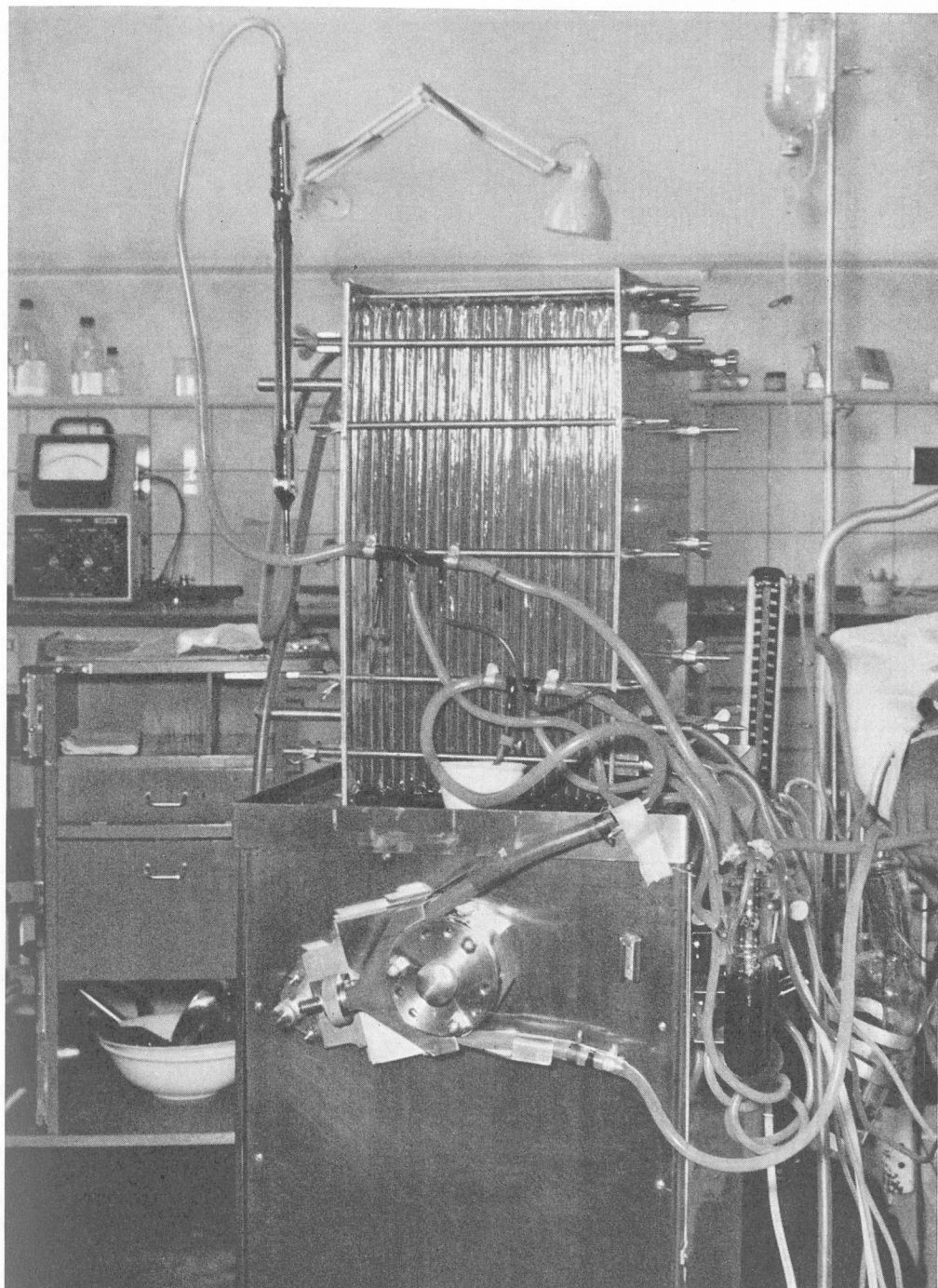
Kommunehospitalets 3. afd. Dialyseafdelingens hæmodialysator («den kunstige nyre»)
