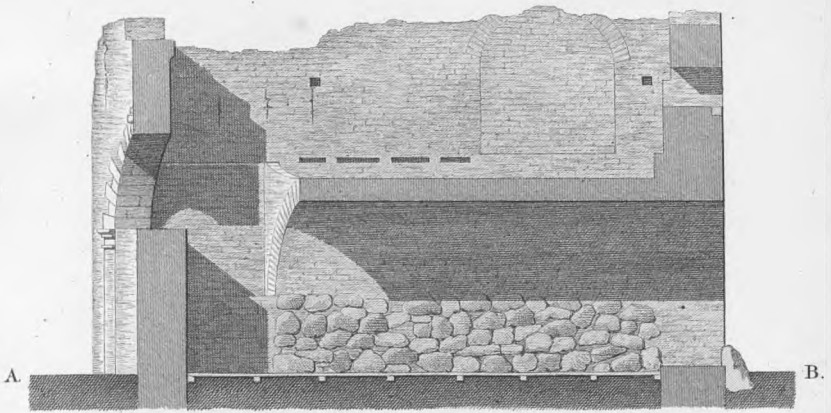
Gjennemsnit mod Nord.
