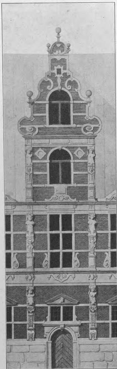
Efter H. C. Ambergs Opmaaling af Børsens nordre Façade
