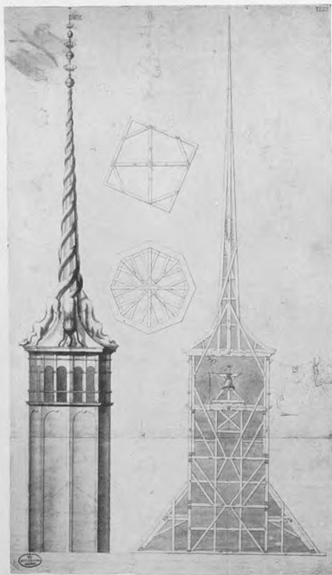
Gl. Tegning af Børsens Taarn og Spir. Nationalmuseet.
