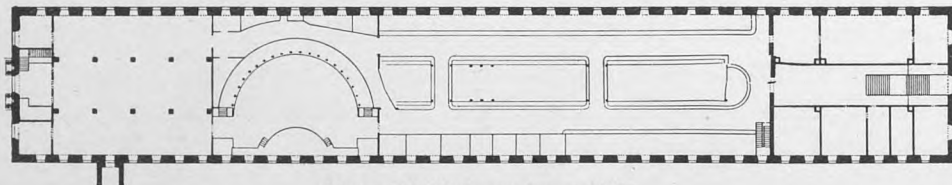
Børsens 1ste Etage som den var 1855.
