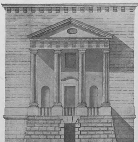
Harsdorffs Udkast (1785) til »Dekorationen« paa Bankbygningens Façade mod Slotspladsen.
