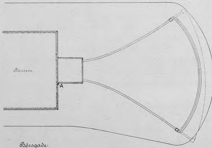
Plan af Børsrampen i dens ændrede Skikkelse.
