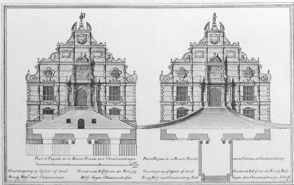
Børsens østre og vestre Gavl. Efter Den danske Vetruvius.
