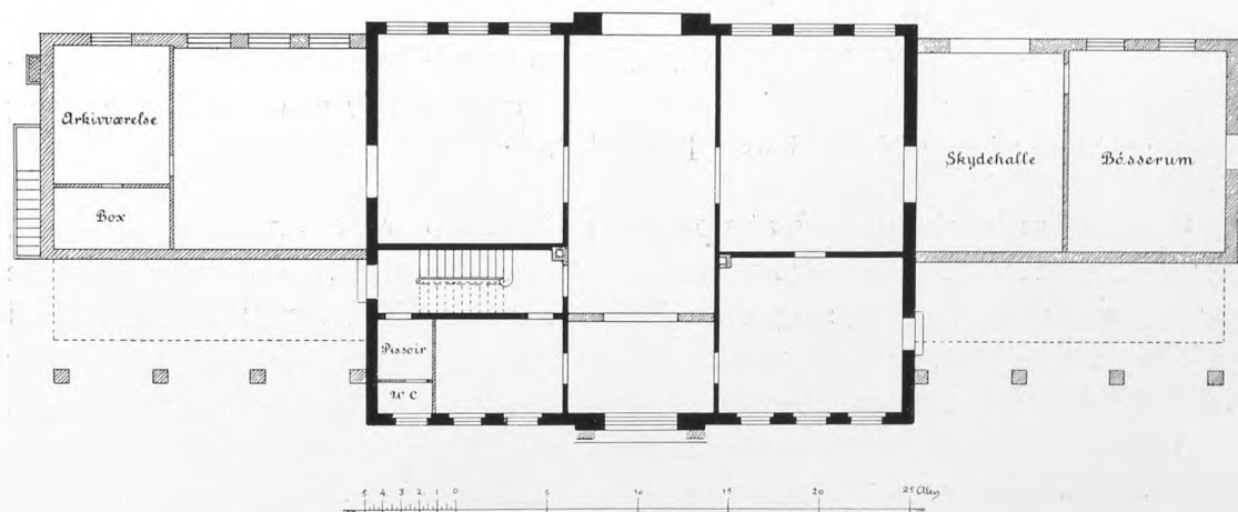
PLAN AF SKYDEHUSET
