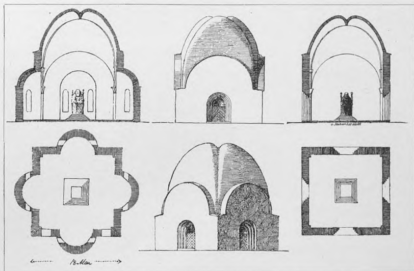
P. V. Jensen Klint: To Udkast til Grundtvigs Mindehal.
