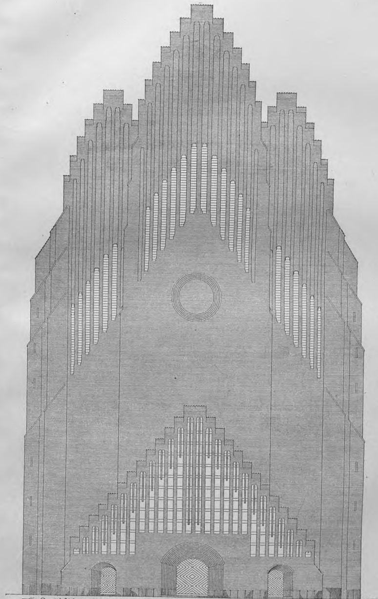
Den 16 de Sept. 1821 GRUNDTVIGS-KIRKECARN: VESTFRONTEN. P. W. Jørgensen's Arkitekt.
