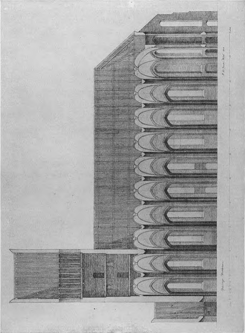
P. V. Jensen-Klint: Længdesnit af Grundtvigs Kirken, 1913,
