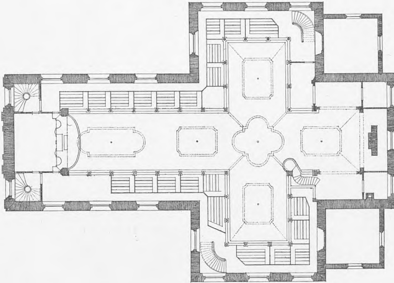
10. Opmaaling af Garnisons Kirke. Loftsplan.
