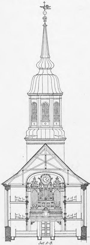
14. Opmaaling af Garnisons Kirke. Snit af Langskibet.
