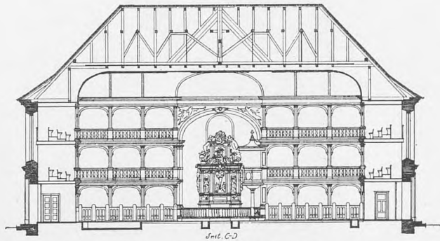
15. Opmaaling af Garnisons Kirke. Snit gennem Choret og gennem Tværskibet.
