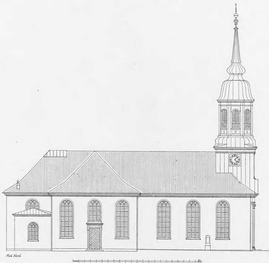
13. Opmaaling af Garnisons Kirke. Nordsiden.
