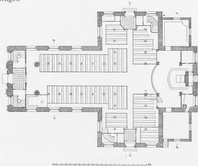
9. Opmaaling af Garnisons Kirke, 1928. Grundplan.
