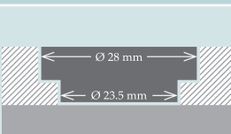
Prindere flanșă - Ø 28 mm
