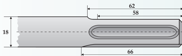
Daltă cu canal
