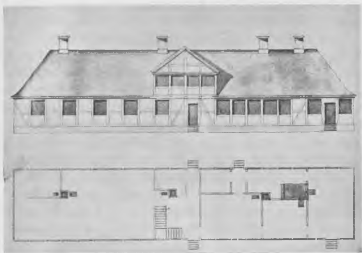
Fig. 2. Tegning til et nyt Gartnerhus paa Frederiksdal efter Generalbygmester E. D. Häussers Forslag 1741. Efter Originaltegning i Rigsarkivet. (Rentek. Sjæll. Stifts Kontors kgl. Resol. 1741. Nr. 2 [12/1]).
