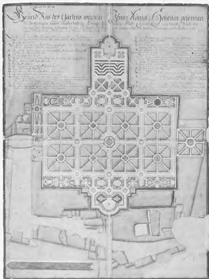
Scheels Forslag til Frederiksberg Haves Anlæg, udført efter 4. August 1697. Planen findes i den historiske Vaabensamling, Artilleriets Tegnearkiv.
