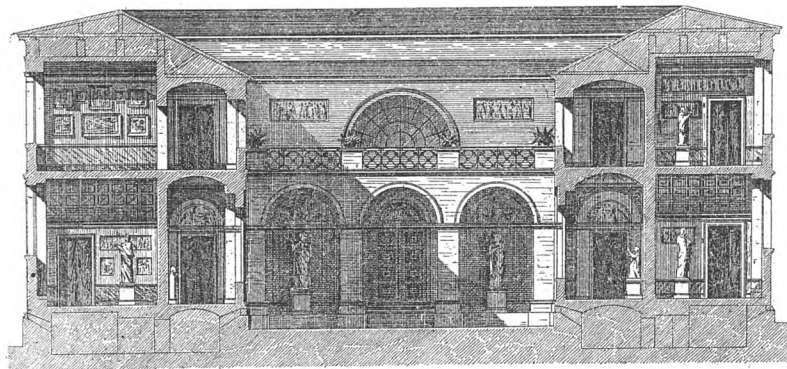
TVÆRSNIT
