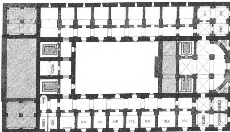
PLAN AF KÆLDEREN
