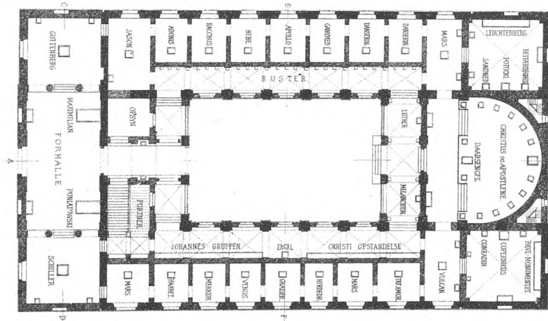
PLAN AF STUEN
