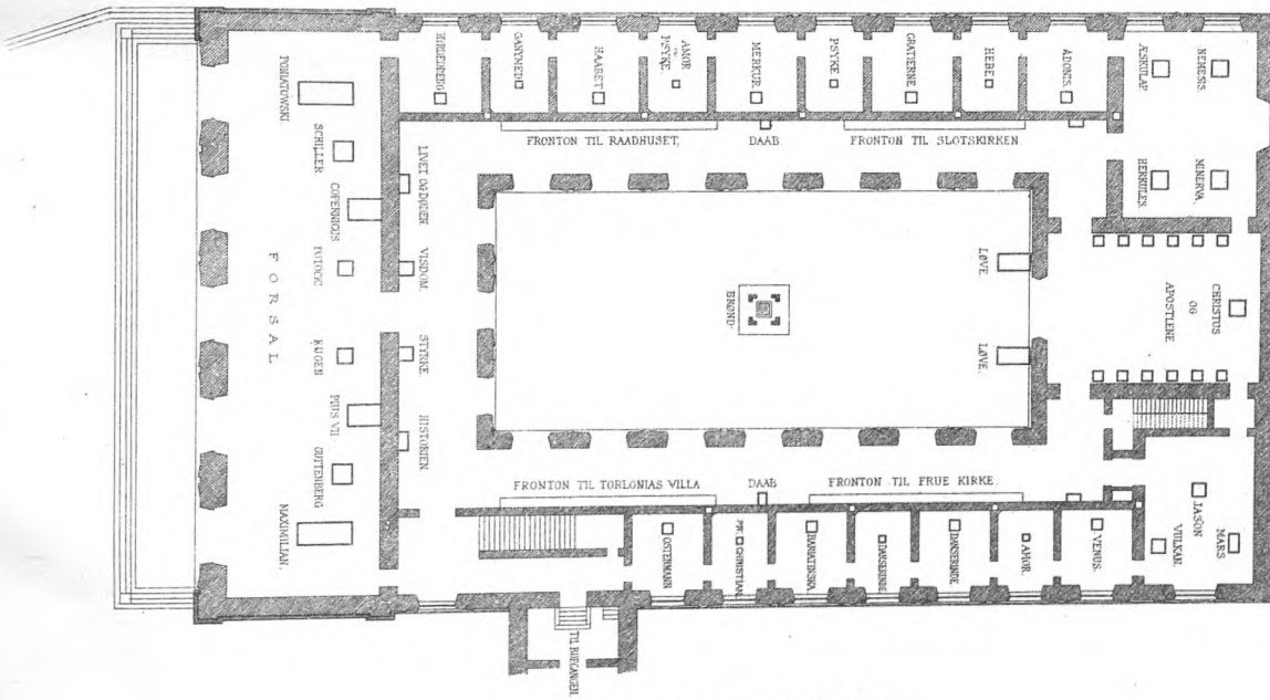
PLAN AF STUEN
