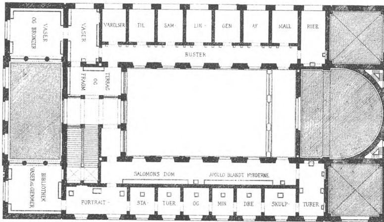
PLAN AF 1 STE SAL
