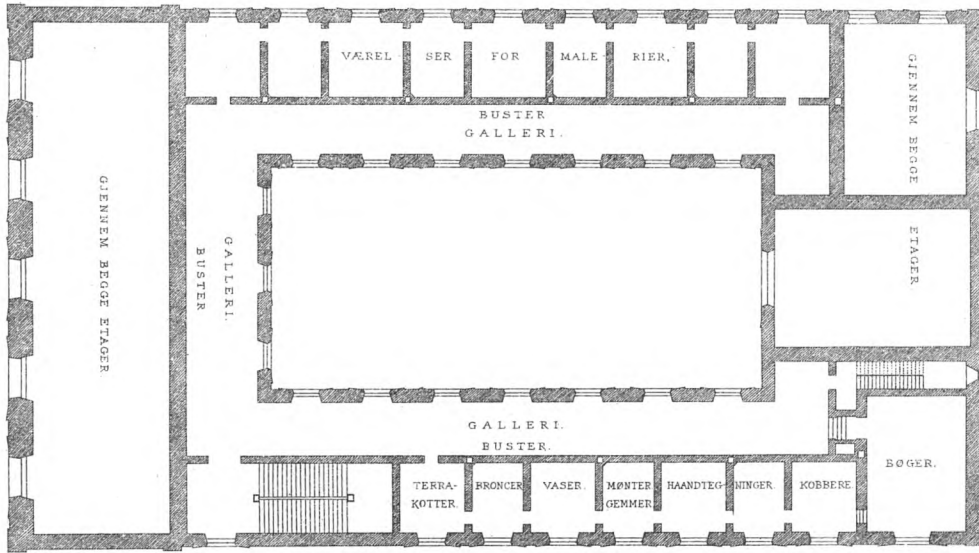
PLAN AF 1STE SAL
