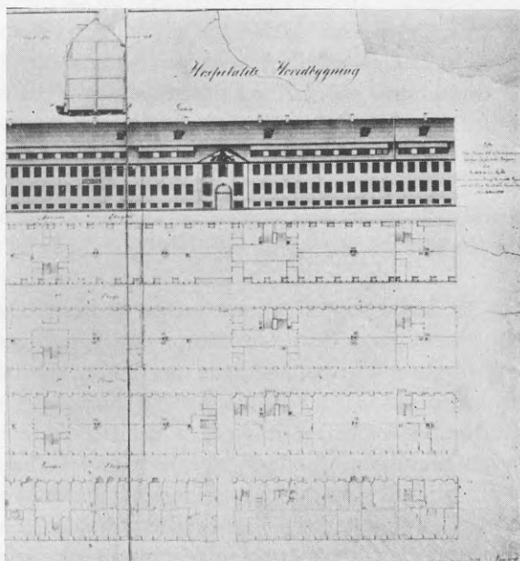
Fig. 22. Garnisonshospitalets hovedbygning. Etage-inddeling.
