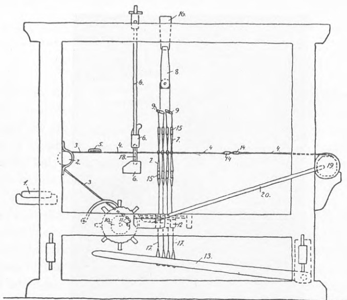
Fig. 9. Skematisk fremstilling af væv. Efter arkitekt H. Zangenberg. 1 Væverens sæde (siddefjæl). 2 Brystbom. 3 Det vævede tøj. 4 Kæden (trendegarnet). 5 Sprøde, der holder tøjet udspændt på tværs. 6 Slagbord. 7 Sølleskafter. 8 Ophængning til rulle eller trisser. 9 Vipper eller nikkepinde. 10 Underløber eller tøjbom med rille (11) til en svibe. 12 Sideheste eller dværsler. 13 Fodskamler. 14 Skelkæppe. 15 Søllekæppe. 16 Søllestang. 17 Snore fra dværsler til fodskamler. 18 Væveskeen eller kammen i slagbordet. 19 Garnbommen. 20 Sidestokken 102 ).
