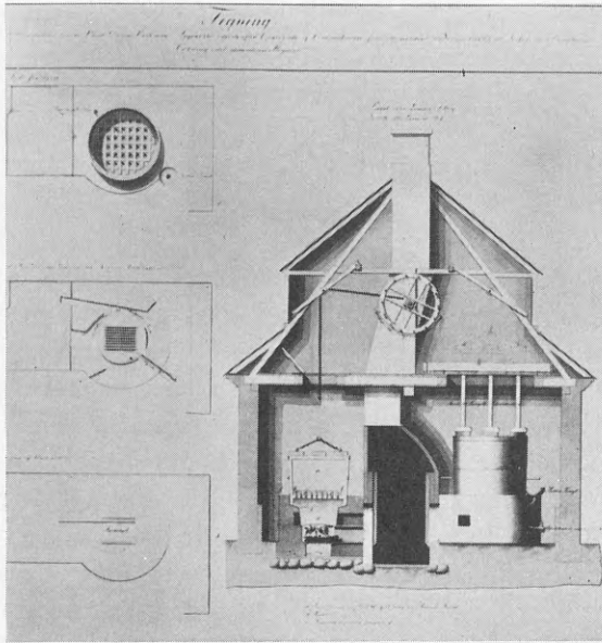
Fig. 23. »Tegning over de 1824 indrettede tvende Vand-Damp-Vaskningsapparater udført efter Opgivelse af Kommissionen, som allernådigst har været befalet til Forslag med Vand-Damp-Vaskning på Almindeligt Hospital«.
