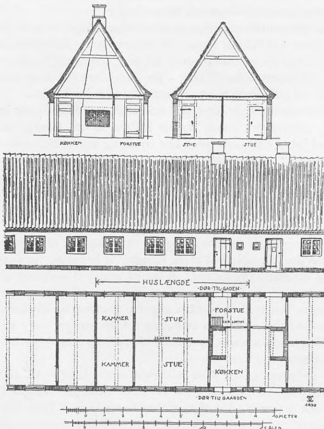
Fig. 31. Opmåling af et af Nyboderhusene med dele af nabohusene i Chr. IV's længe i St. Paulsgade.
