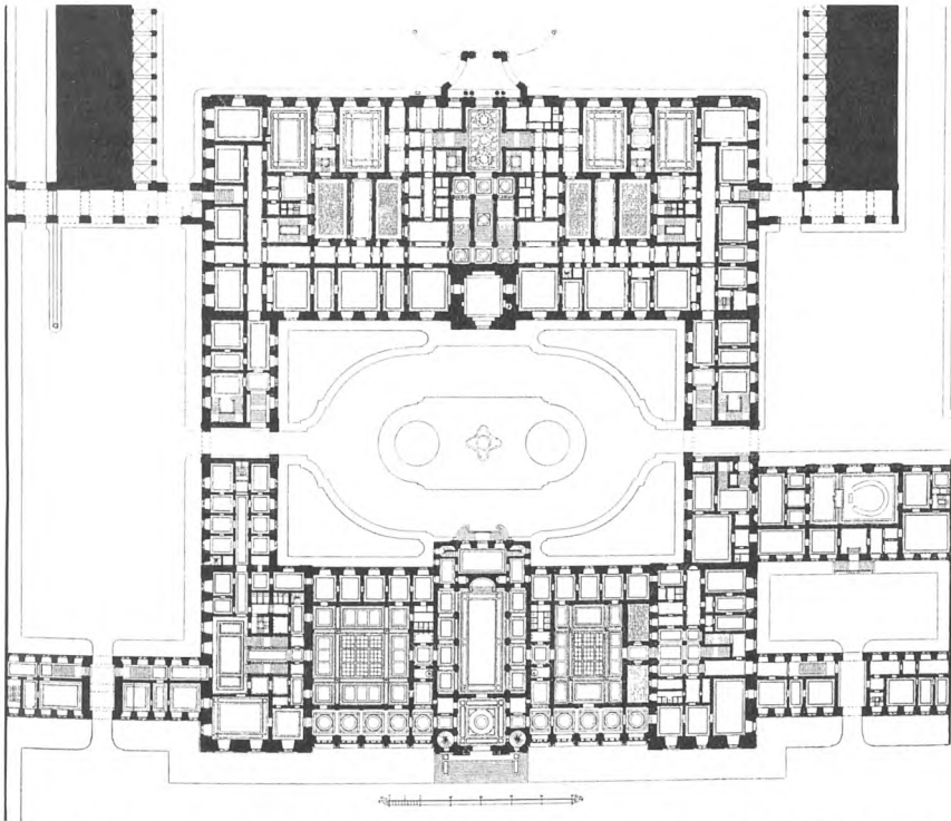
FIG. 44. PROJEKT TIL CHRISTIANSBORG SLOTS GENOPFØRELSE. 1888. PLAN AF DAMEETAGEN. ARCHITEKT MARTIN BORCH.
