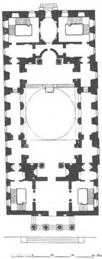
FIG 10. CHRISTIANSBORG SLOT. PLAN AF SLOTSKIRKEN. ARCHITEKT C. F. HANSEN.
