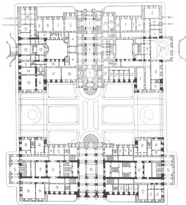
FIG. 38. PROJEKT TIL CHRISTIANSBORG SLOTS GENOPFØRELSE. 1887. PLAN AF DAMEETAGEN. ARCHITEKT F. T. E. BLICHFELDT.
