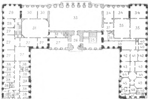
FIG. 56. PLAN AF KONGEFLOJENS KONGEETAGE.
