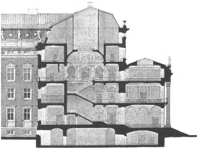
FIG. 73. PROJEKT TIL CHRISTIANSBORG SLOTS GENOPFØRELSE. 1897. SNIT GENNEM RIGSDAGSFLOJENS MIDTPARTI. ARCHITEKT ALBERT JENSEN.
