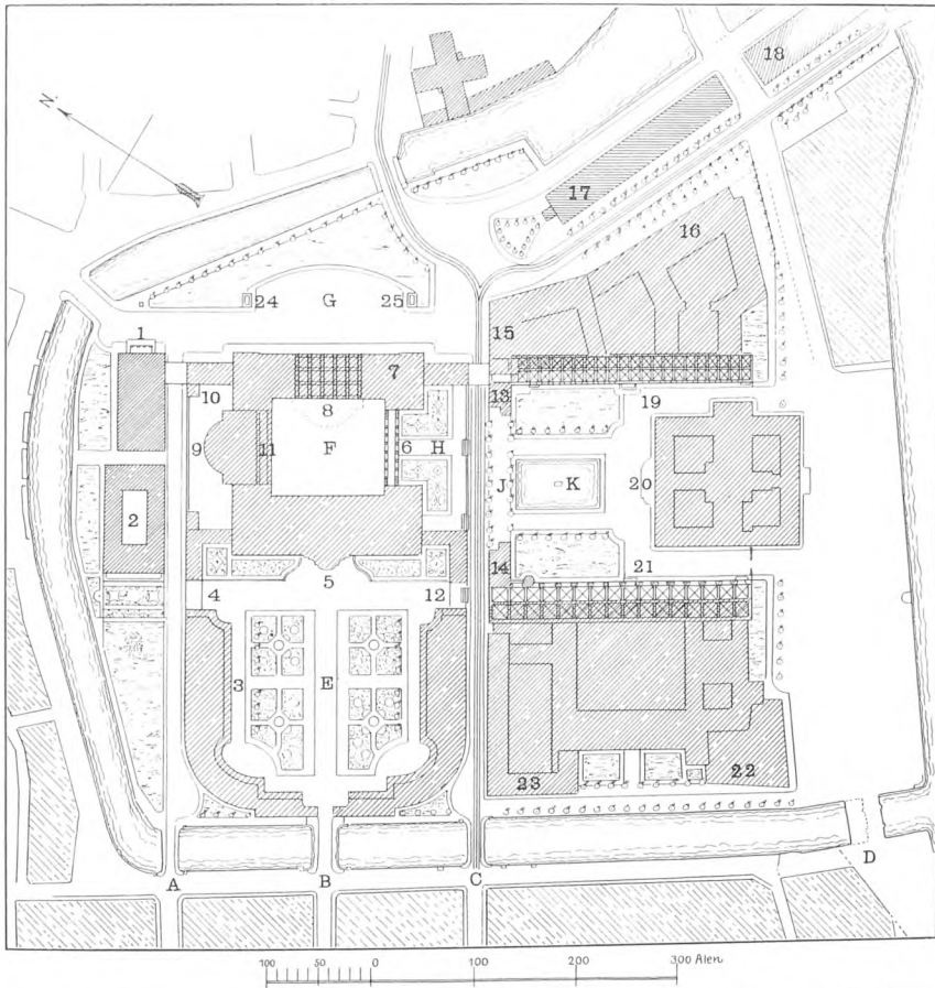
FIG. 80. PROJEKT TIL SLOTSHOLMENS REGULERING. 1898. ARCHITEKTER P. KROHN OG M. NYROP. A. Stormbroen. B. Marmorbroen. C. Prindsens Bro D. Havnebanebroen. E. Ridebanen. F. Slotsgaarden. G. Slotspladsen. H. Kavalergaarden. J. Den nedbrudte Del af store kgl. Bibliothek. K. Vandbassin i gamle Tøjhusgaard. 1. Slotskirken. 2. Thorvaldsens Museum. 3. Ridehuset. 4. Gennembrydning af Buegangen. 5. Slotsløj mod Ridebanen. 6. Ny Kolonnade mod Kavalergaarden. 7. Højesteret. 8. Ny Hovedport mod Slotspladsen. 9. Rigsdags-salene. 10. Klokketaarn for Slotskirken. 11. Eventuel Kolonnade mod Prinds Jørgens Gaard. 12. Gennembrydning af Buegangen mod Tøjhuset. 13. 14. Bevarede Dele af gamle store kgl. Bibliothek. 15. Kancellibygningen. 16. Den Lercheske Gaard. 17. Børsen. 18. Nybørs. 19. Proviantgaarden. 20. Det nye store kgl. Bibliothek. 21. Lange Tøjhus. 22. Gamle Bryghus. 23. Staldmestergaarden. 24. 25. Rytterstatuer.
