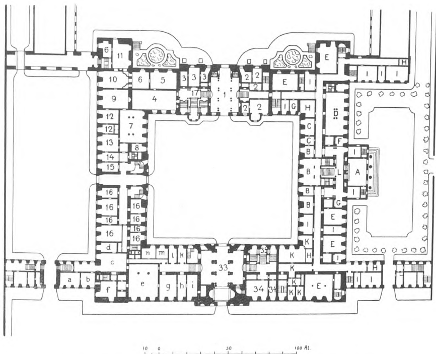
FIG. 77. PROJEKT TIL CHRISTIANSBORG SLOTS GENOPFØRELSE. 1897. PLAN AF DAMEETAGEN. ARCHITEKT ALBERT JENSEN.
