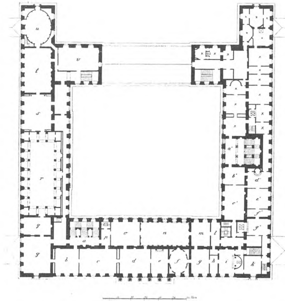
FIG. 4. CHRISTIANSBORG SLOT. KONGENS ETAGE. ARCHITEKT C. F. HANSEN.
