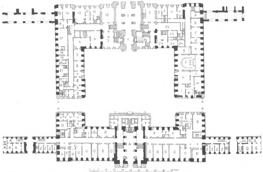
FIG. 55. PROJEKT TIL CHRISTIANSBORG SLOTS GENOPFØRELSE. 1888. PLAN AF DAMEETAGEN. ARCHITEKT H. C. AMBERG.
