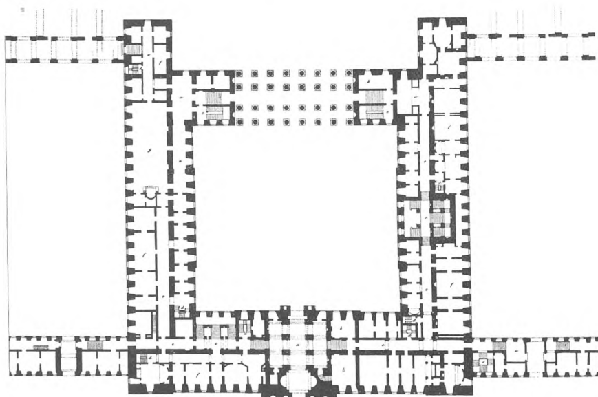
FIG. 3. CHRISTIANSBORG SLOT. DAMEETAGEN. ARCHITEKT C. F. HANSEN.
