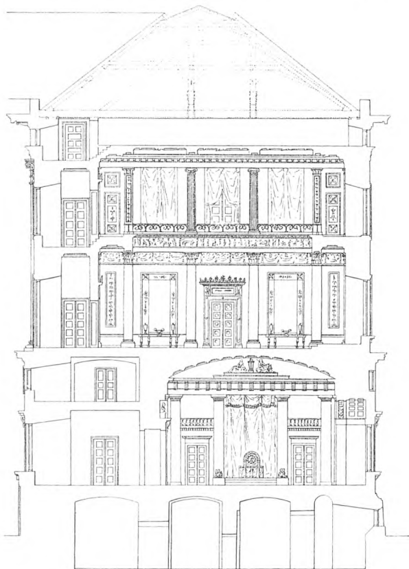
FIG. 8. CHRISTIANSBORG SLOT. SNIT GENNEM SIDEFLOJEN MED RIDDERSALEN OG HØJESTERETSSALEN. ARCHITEKT C. F. HANSEN.
