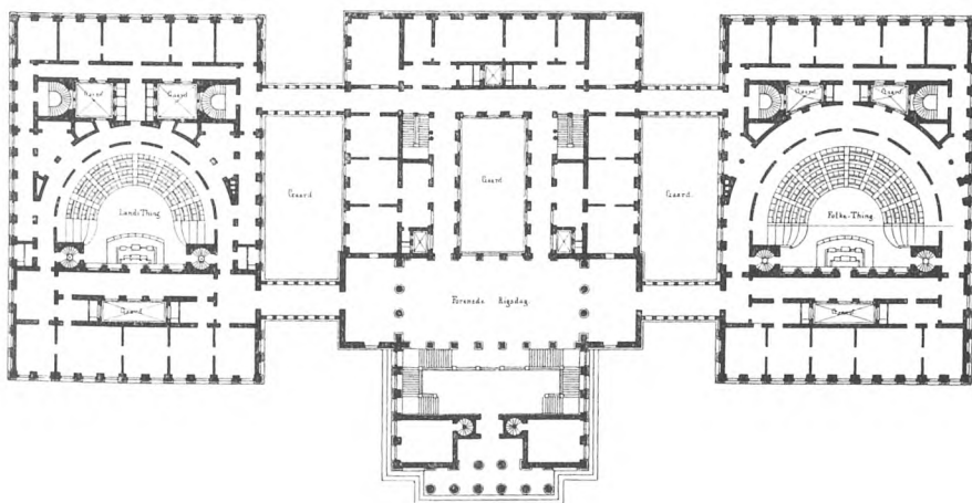
FIG. 20. PROJEKT TIL EN RIGSDAGSBYGNING I CHRISTIANSGADE. 1884. ARCHITEKT THEOPHILUS HANSEN.
