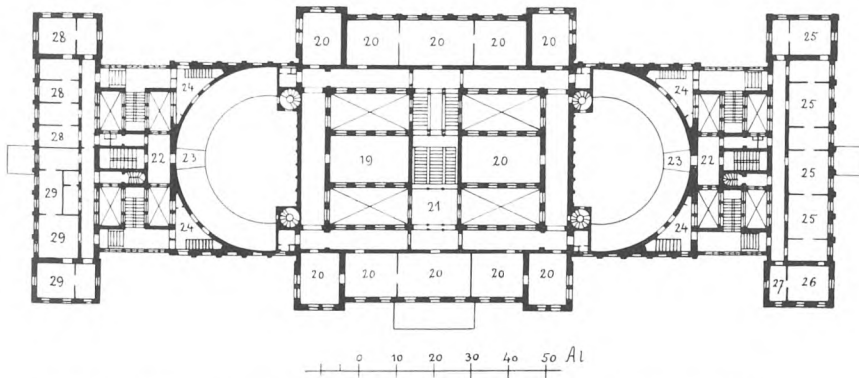
FIG. 24. PROJEKT TIL EN RIGSDAGSBYGNING I CHRISTIANSGADE. 1886. HOVEDETAGEN. ARCHITEKT THEOPHILUS HANSEN.
