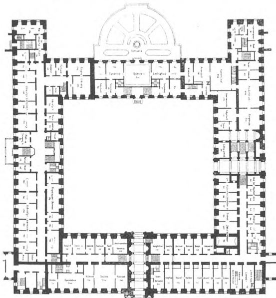
FIG. 65. PROJEKT TIL CHRISTIANSBORG SLOTS GENOPFØRELSE. 1894. PLAN AF DAMEETAGEN. ARCHITEKT J. D. HERHOLDT.
