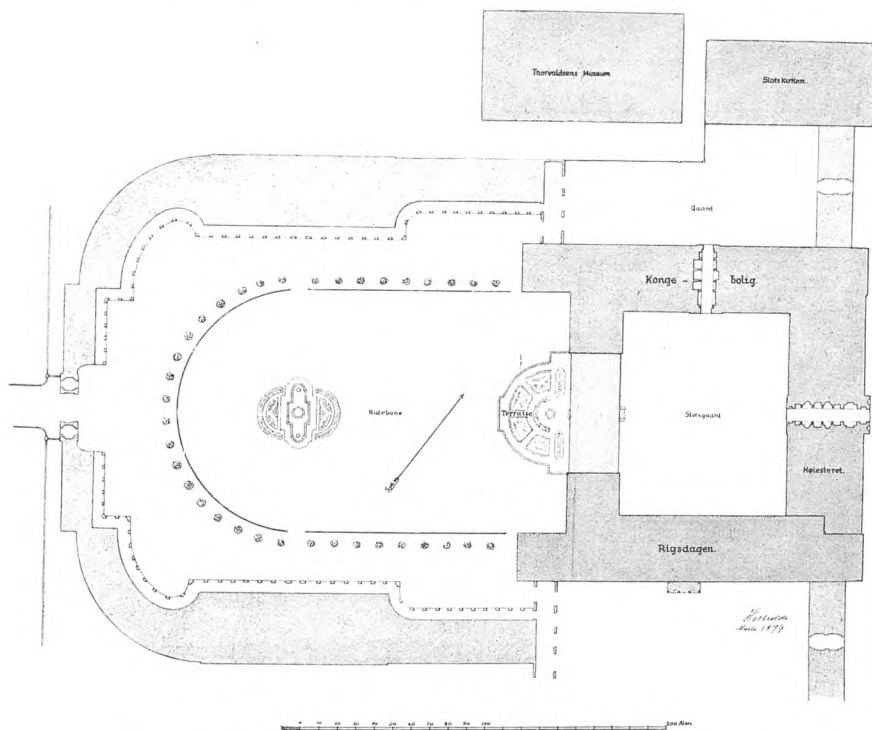
FIG. 64. PROJEKT TIL CHRISTIANSBORG SLOTS GENOPFØRELSE. 1894. OVERSIGTSPLAN. ARCHITEKT J. D. HERHOLDT.
