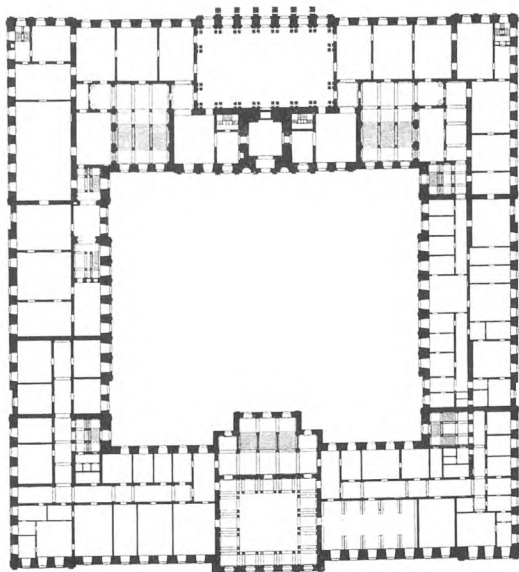
FIG. 51. PROJEKT TIL CHRISTIANSBORG SLOTS GENOPFØRELSE. 1888. PLAN AF KONGEETAGEN. ARCHITEKTER O. P. MOMME OG L. F. OLESEN.
