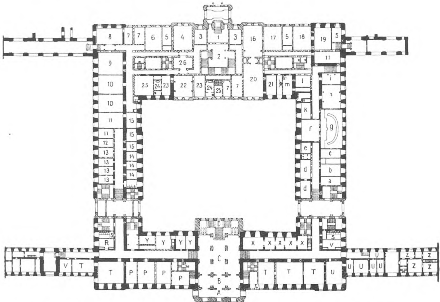
FIG. 61. PROJEKT TIL CHRISTIANSBORG SLOTS GENOPFØRELSE. 1888. PLAN AF DAMEETAGEN. ARCHITEKT L. H. KNUDSEN. *)
