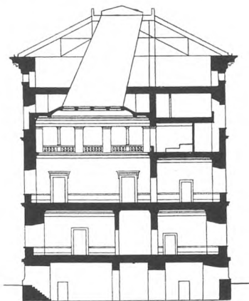
FIG. 68. SNIT GENNEM FOLKETHINGETS LOKALER.
