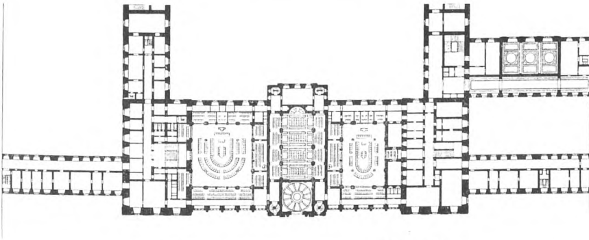
FIG. 46. PLAN AF RIGSDAGSFLØJENS MEZZANINETAGE.
