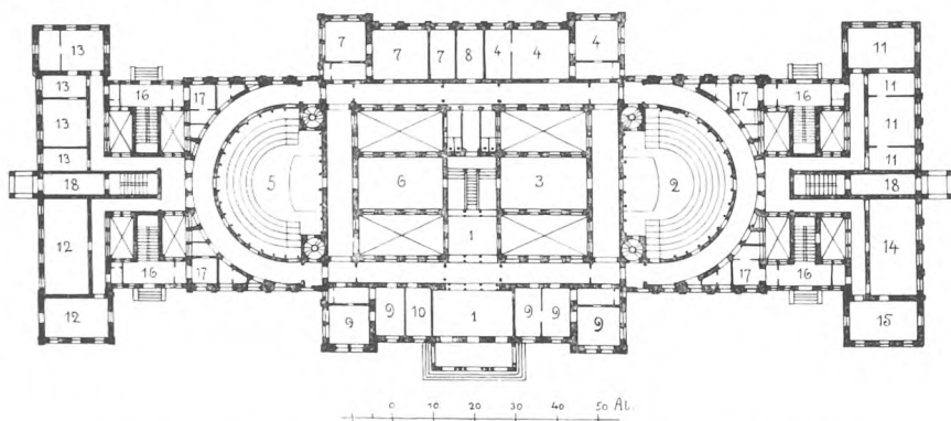
FIG. 23. PROJEKT TIL EN RIGSDAGSBYGNING I CHRISTIANSGADE. 1886. STUEETAGEN. ARCHITEKT THEOPHILUS HANSEN.
