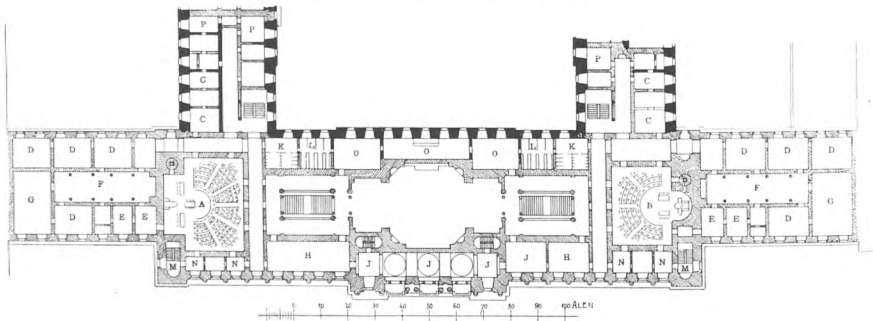
FIG. 34. PLAN AF RIGSDAGSFLØJENS KONGEETAGE.
