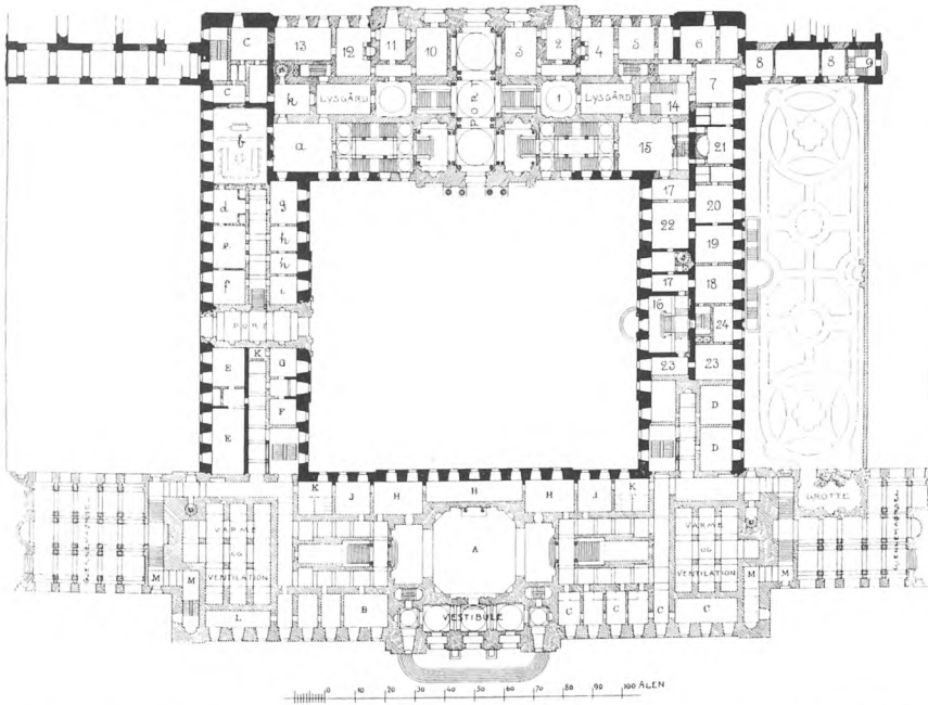
FIG. 30. PROJEKT TIL CHRISTIANSBORG SLOTS GENOPFØRELSE. 1887. PLAN AF DAMEETAGEN. ARCHITEKT L. CLAUSEN.
