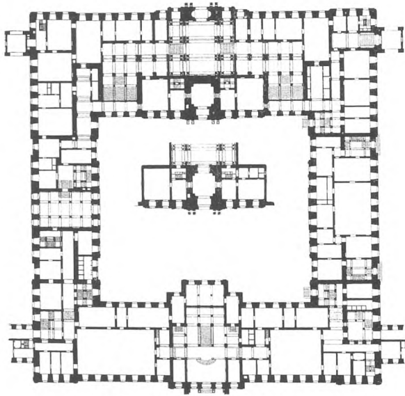
FIG. 50. PROJEKT TIL CHRISTIANSBORG SLOTS GENOPFØRELSE. 1888. PLAN AF DAMEETAGEN. ARCHITEKTER O. P. MOMME OG L. F. OLESEN.
