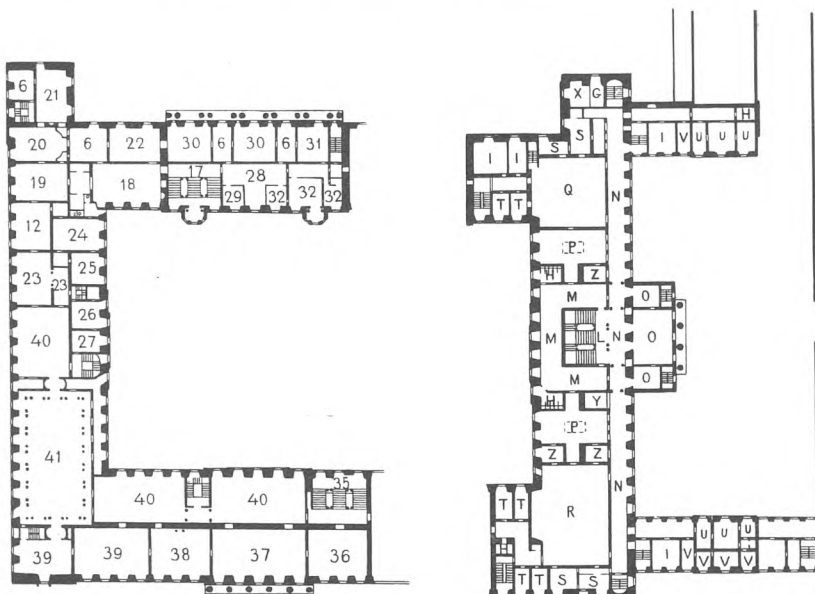
SLOTTETS KONGEETAGE. RIGSDAGENS BELETAGE. FIG. 78-79. PROJEKT TIL CHRISTIANSBORG SLOTS GENOPFØRELSE. 1897. ARCHITEKT ALBERT JENSEN.
