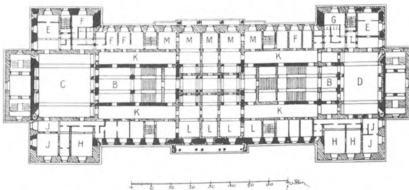
FIG. 40. PLAN AF RIGSDAGSFLOJENS KONGEETAGE.
