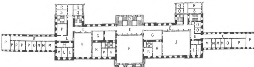
FIG. 63. PLAN AF RIGSDAGSFLØJENS KONGEETAGE.
