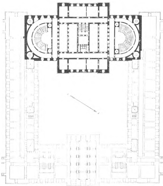
FIG. 21. CHRISTIANSBORG SLOT. PROJEKT TIL RIGSDAGENS ANBRINGELSE I RIDEBANEFLOJEN. ARCHITEKT THEOPHILUS HANSEN.
