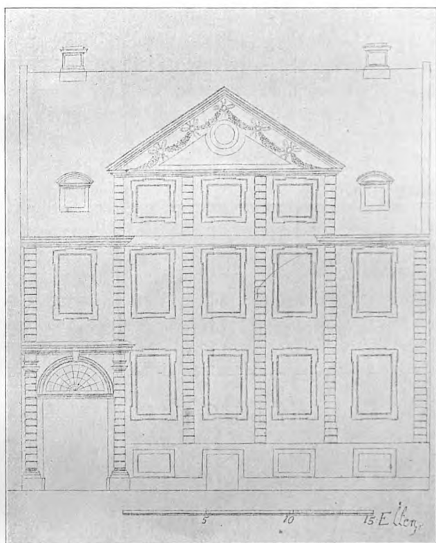
Fig. 6. Typetegning til mere anseligt Borgerhus. (Efter Krieger 1729).
