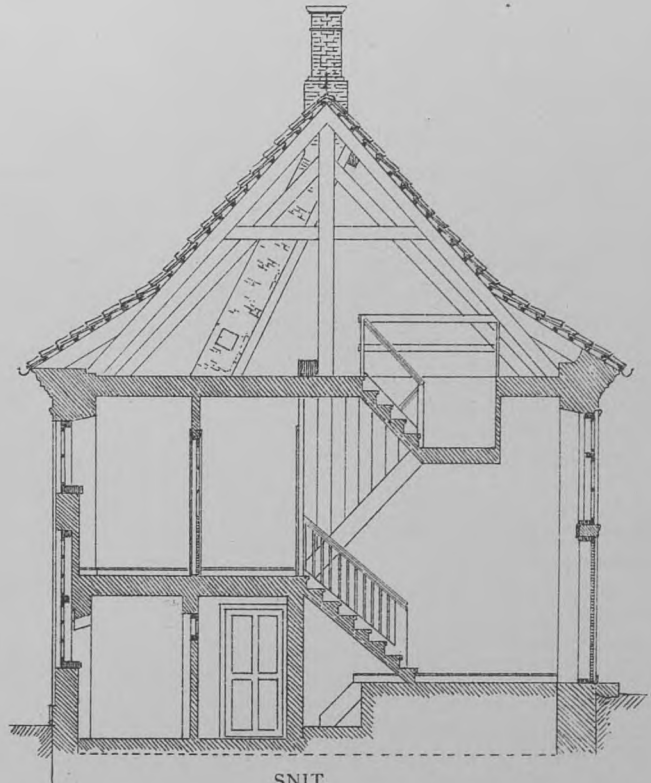
SNIT.
