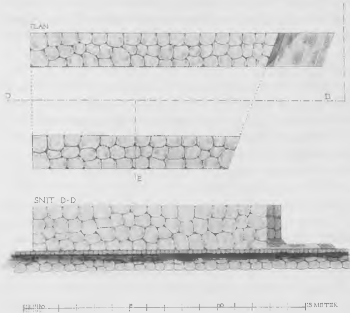
Fig. 3. Plan og Opstalt af Vesterports Mure 1865.
