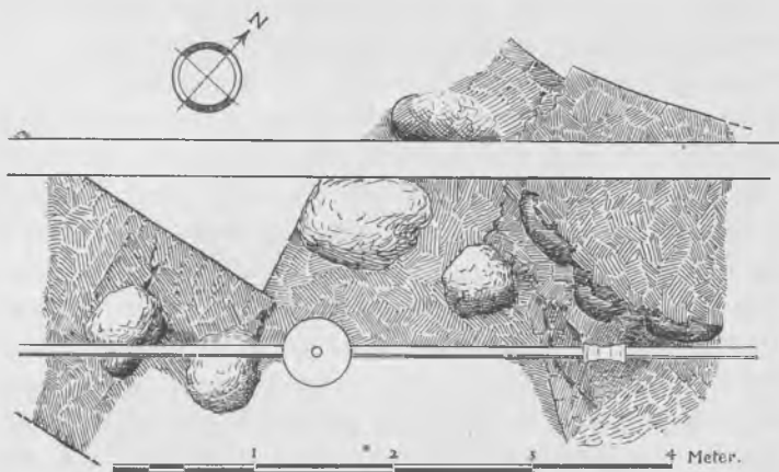
Fig. 2. Detailplan af Fundamenternes søndre Del.
