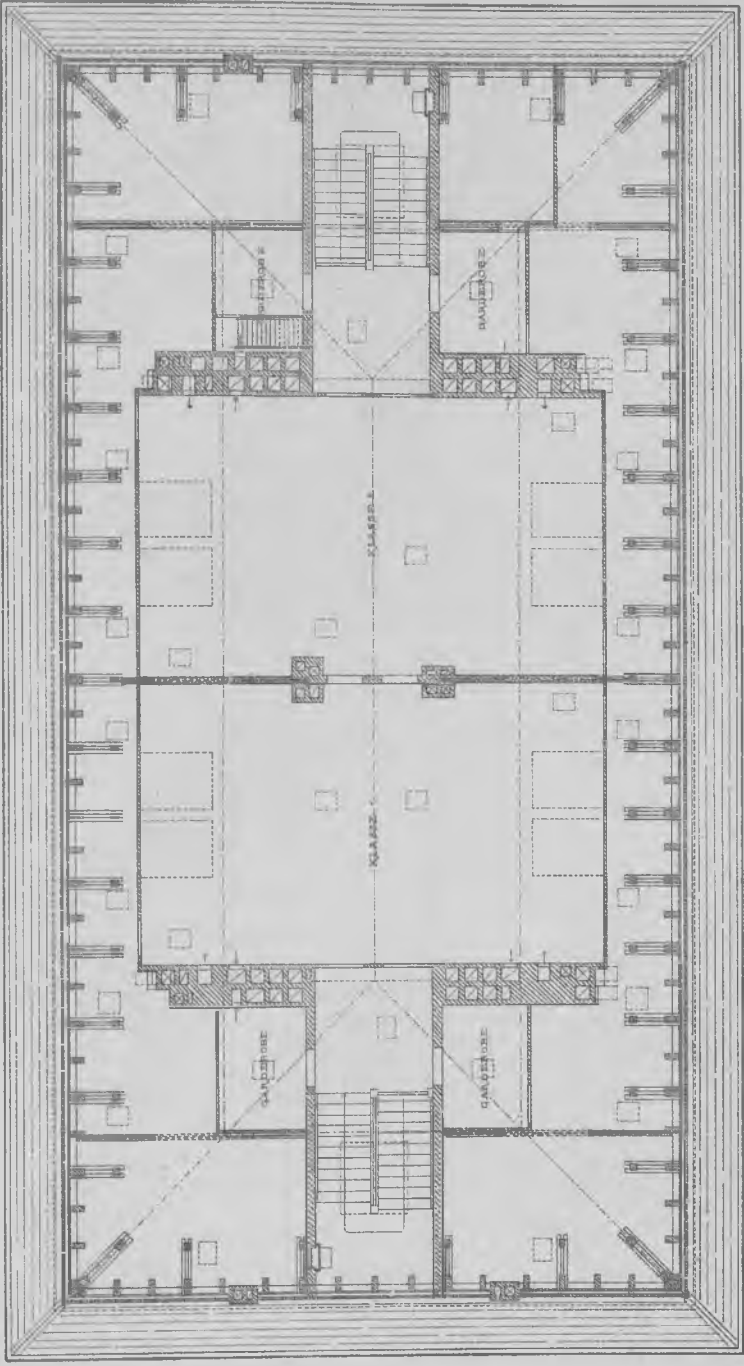
•TAGEPLAN•
