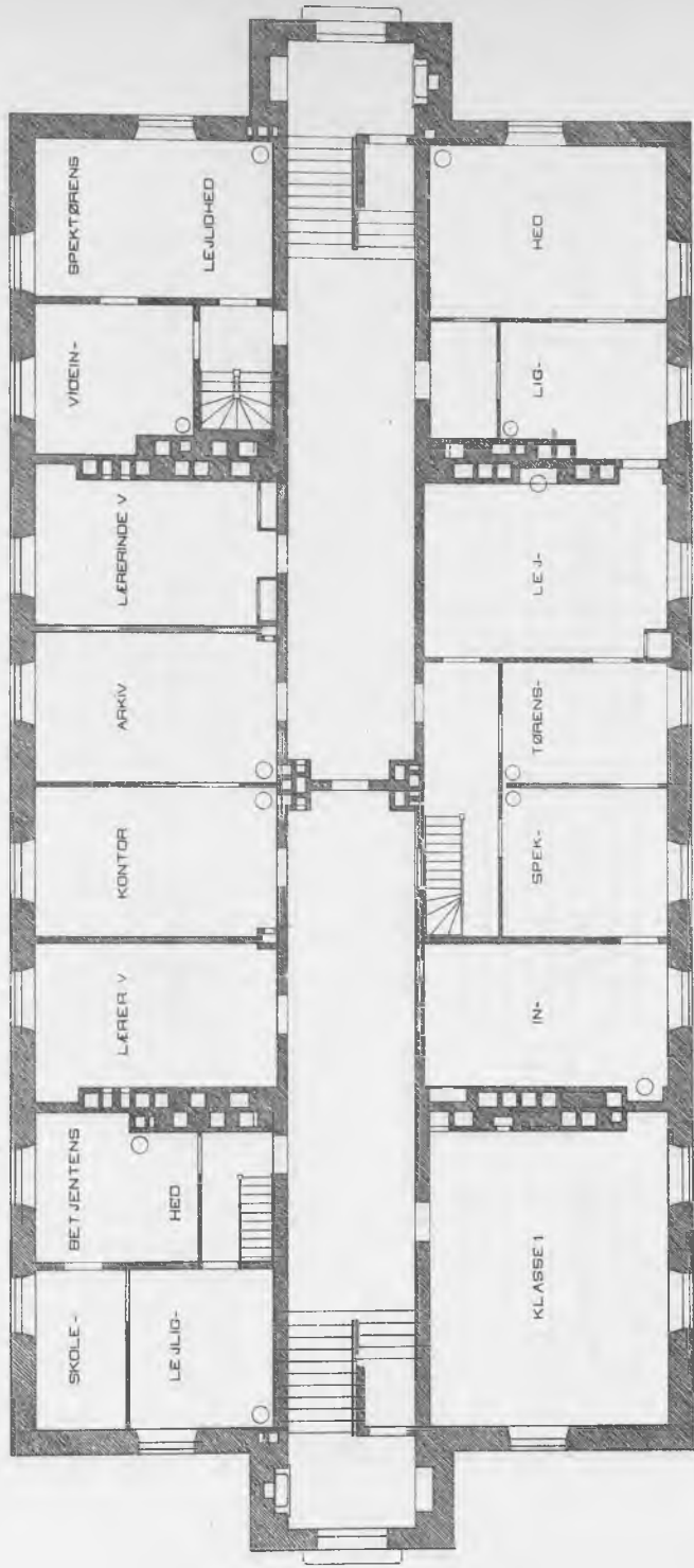
PLAN AF STUEN.
