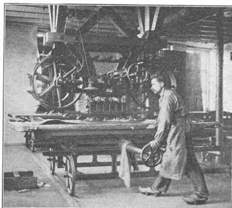
Stødemaskine i Arbejde.
