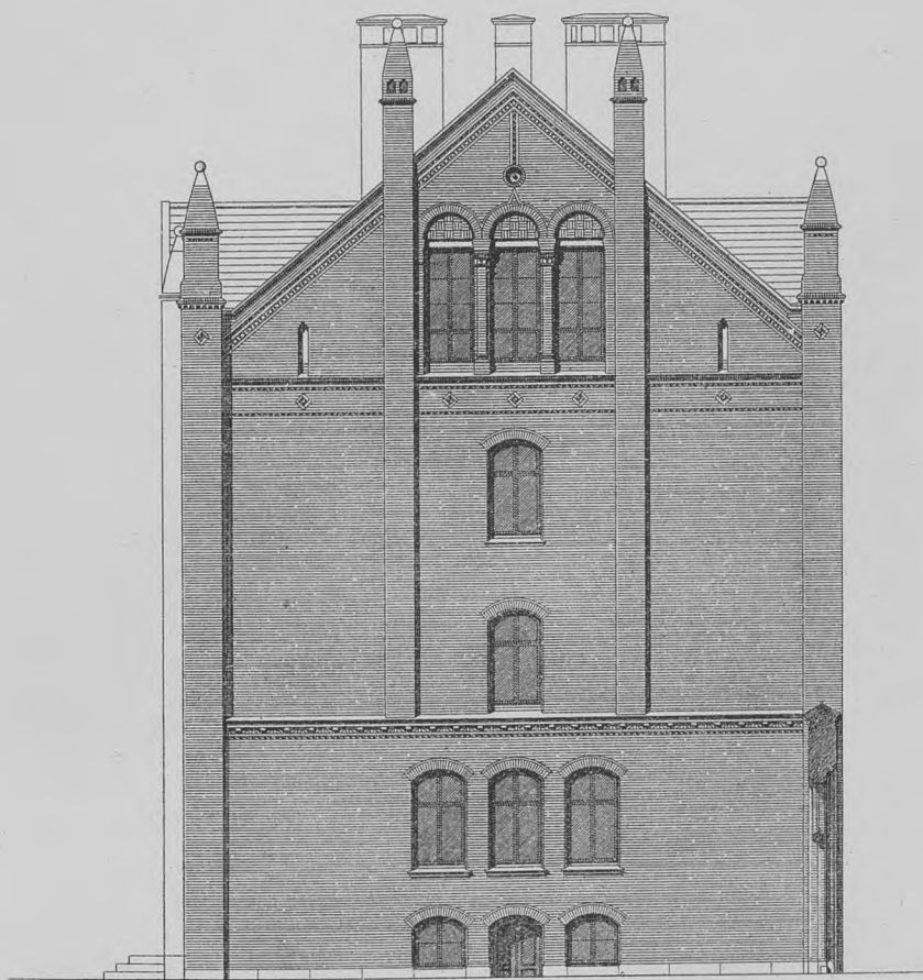
Gavl mod Øst ·
