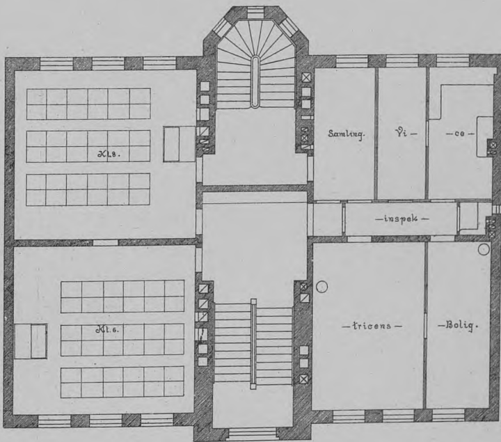
Plan af 1de Sal.
