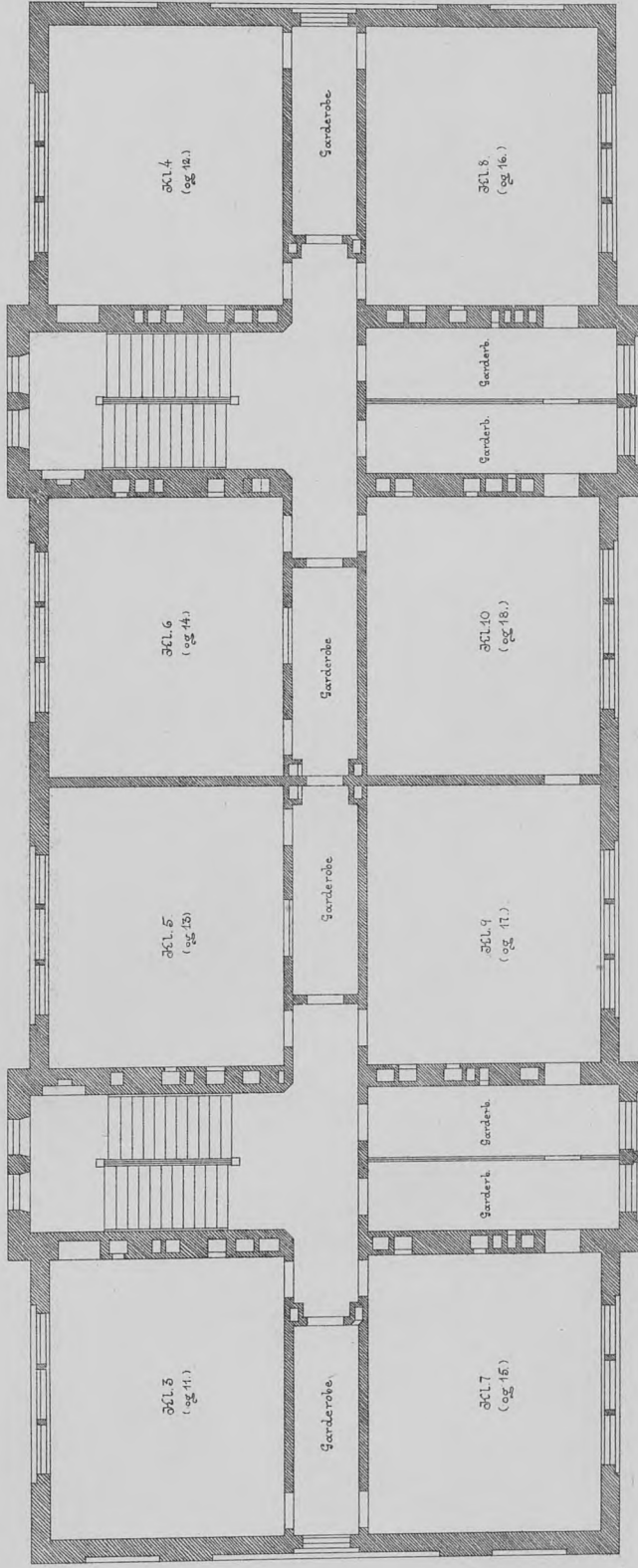
Plan af 1ste Sal. (og 2den Sal.)
