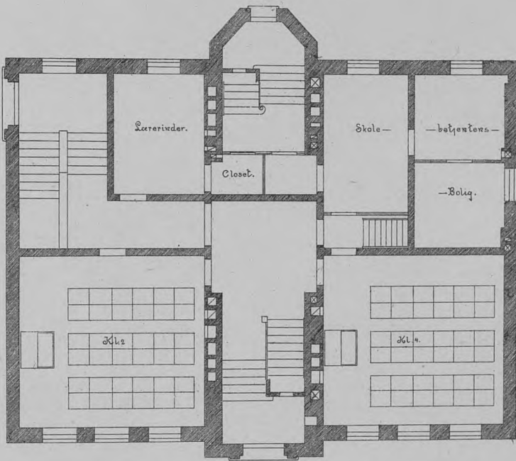
Plan af Stuen.
