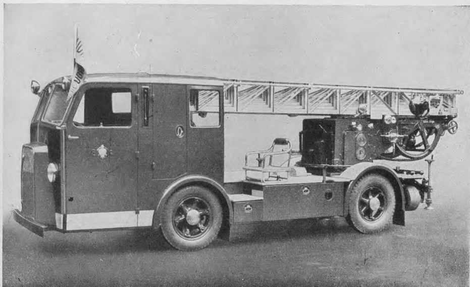
22 m Drejestige. 1939. (Pekingeseren.)
