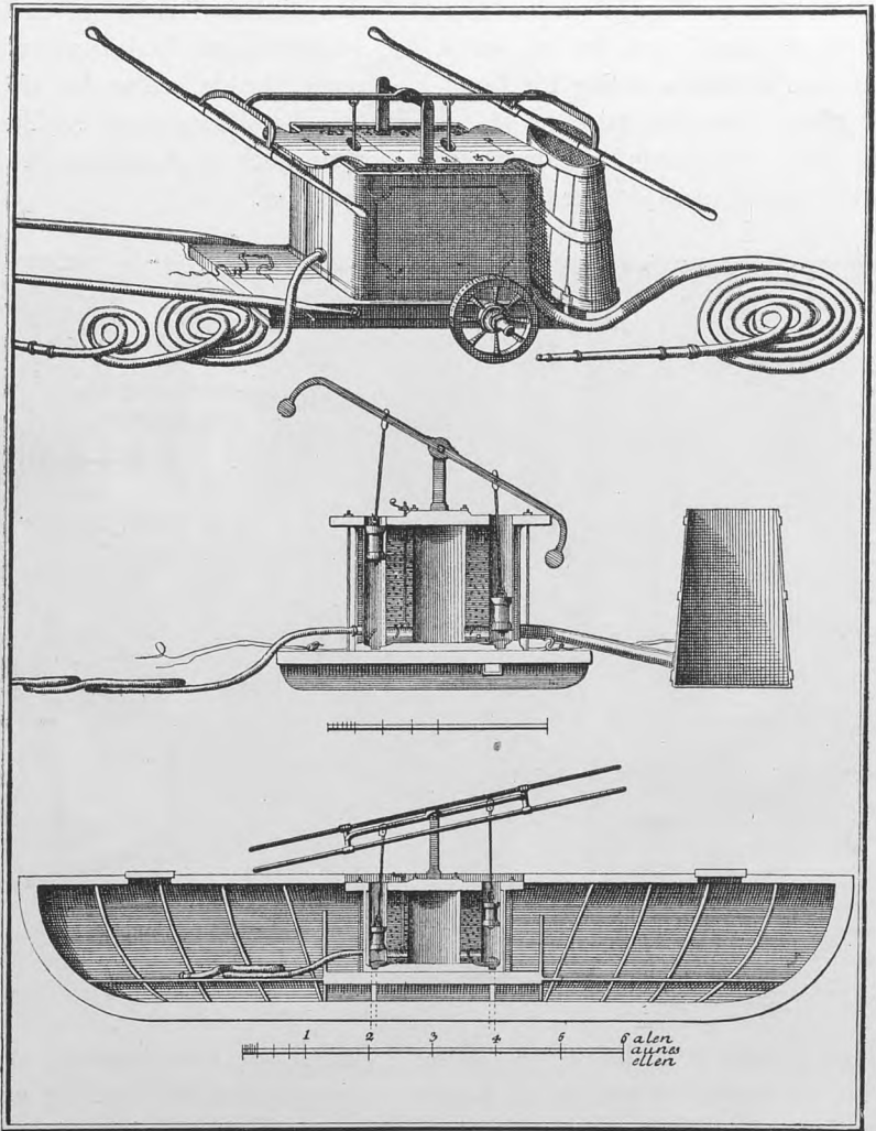
En stor Sprøjte (foroven) og en Pramsprøjte.
