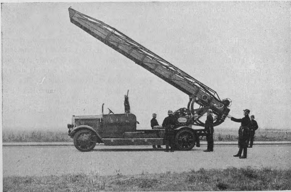
Drejestige, Model 1929, med Stigen rejst.
