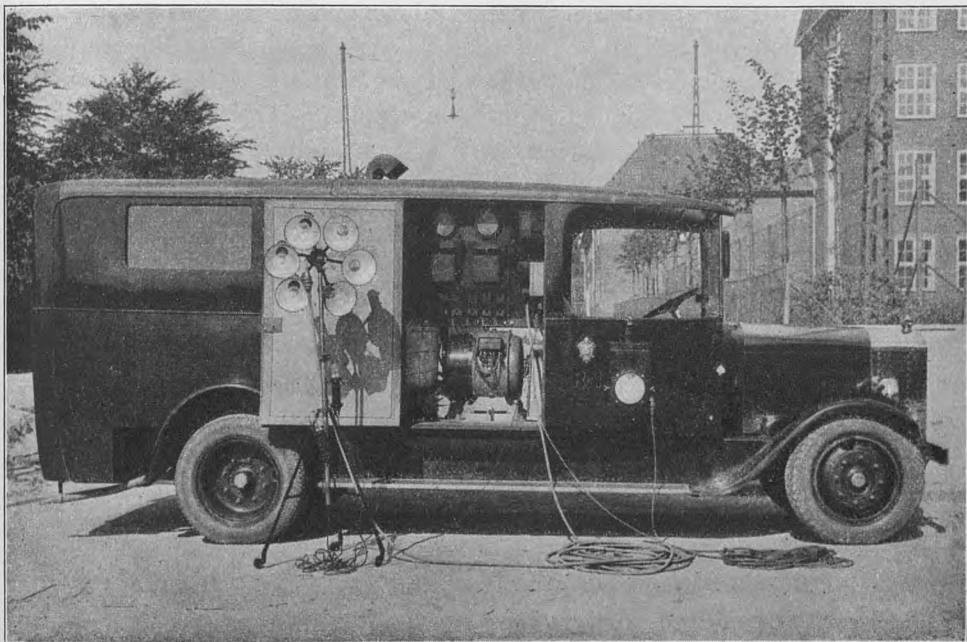
Røgtender Model 1930, set fra Siden med Dynamo og Belysningsmateriel. (Kbh. Brandvæsen)
