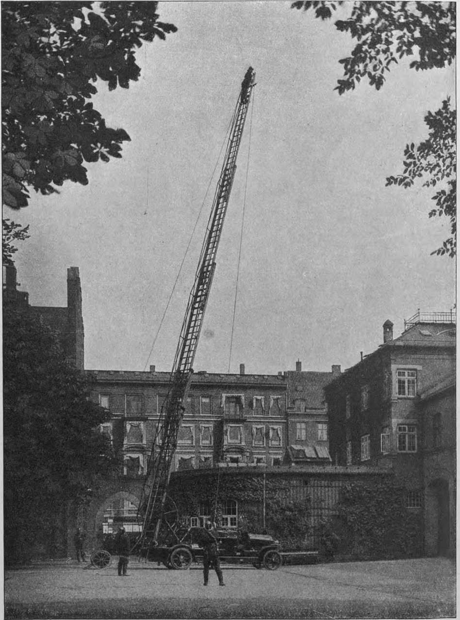
Den elektriske Stige, rejst og udskudt.
