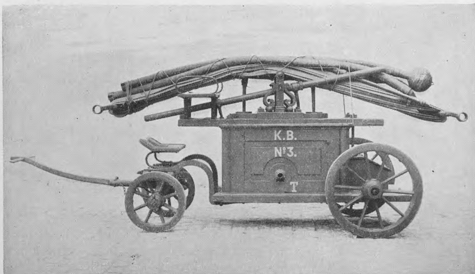
GI. Sprøjte fra Københavns Brandvæsen.
