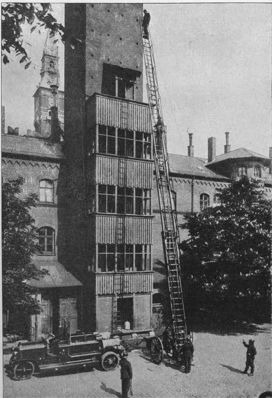
22 m Automobil Afprøvsstige, rejst og udskudt. 1924.
