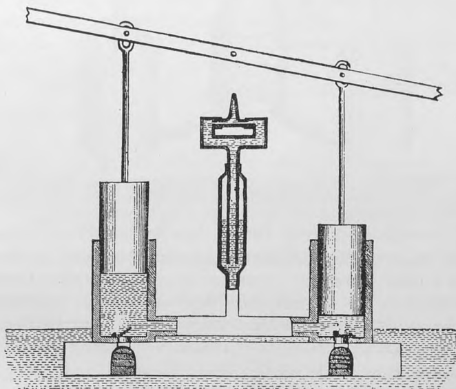
Pumpe efter Beskrivelse i Herons »Pneumatica«, tegnet af Vitruvius.
