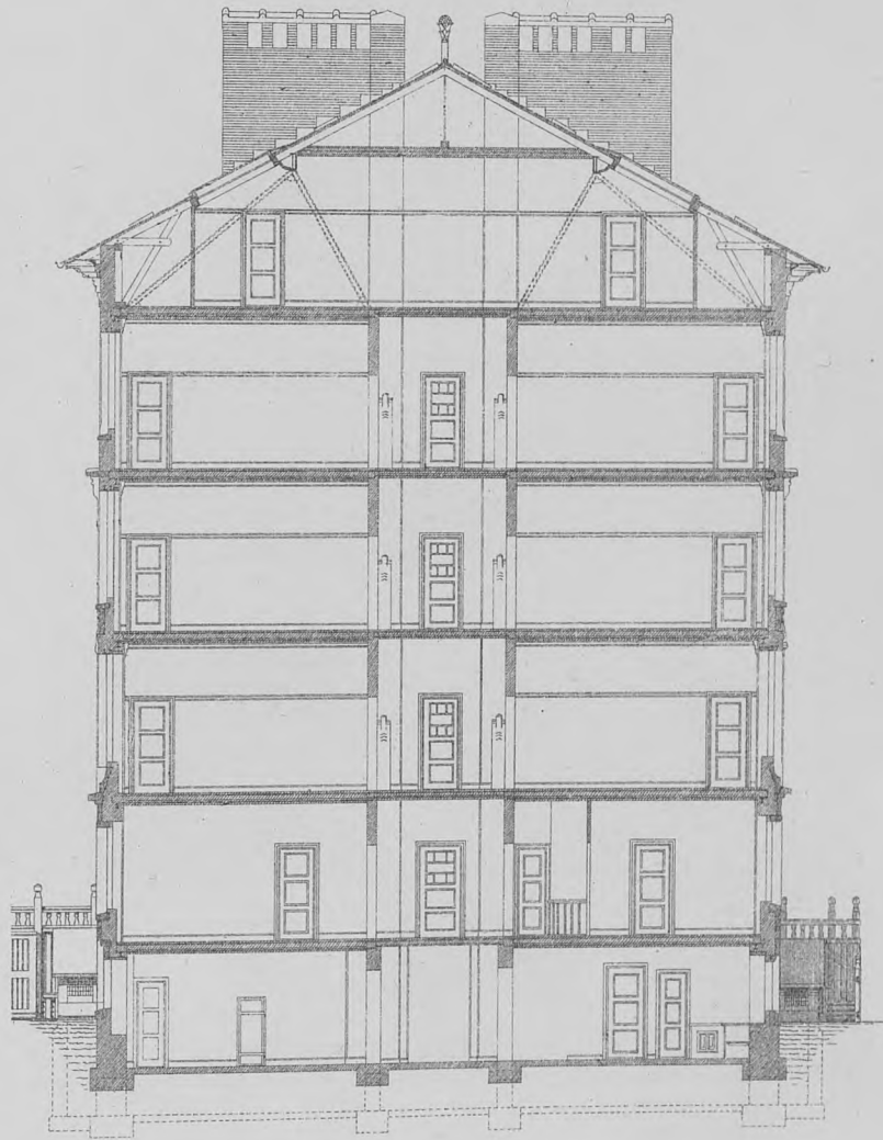
Snit A-B.
