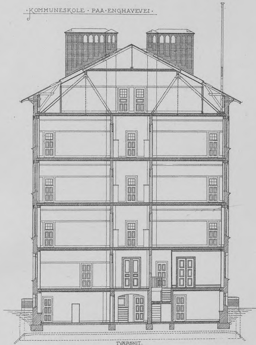
TVÆRSNIT.
