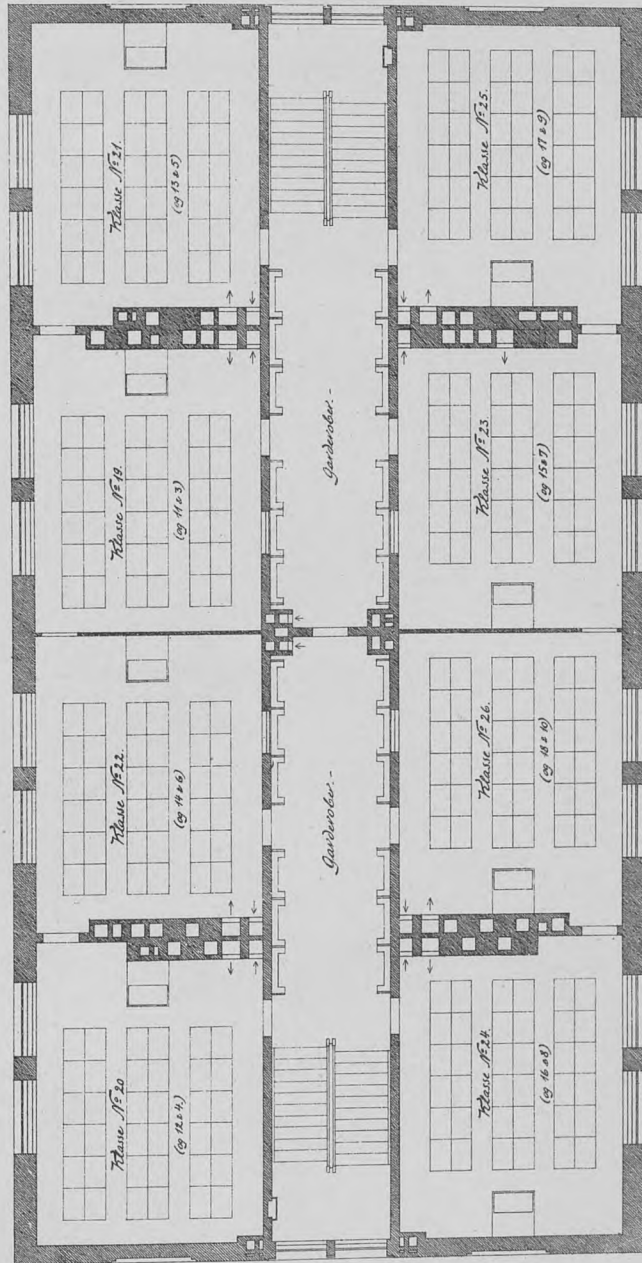
Plan af 1 o (22-25) Sal.
