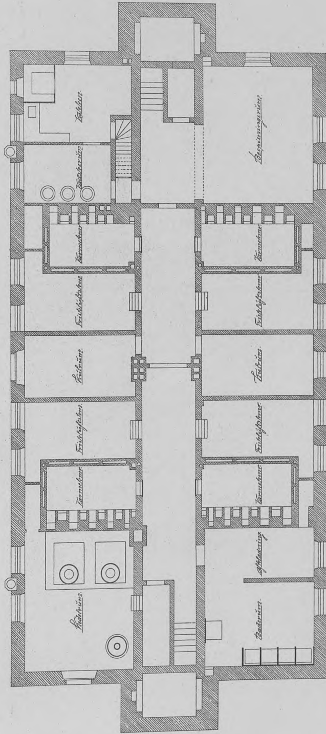
• KJELDERPLAN •
