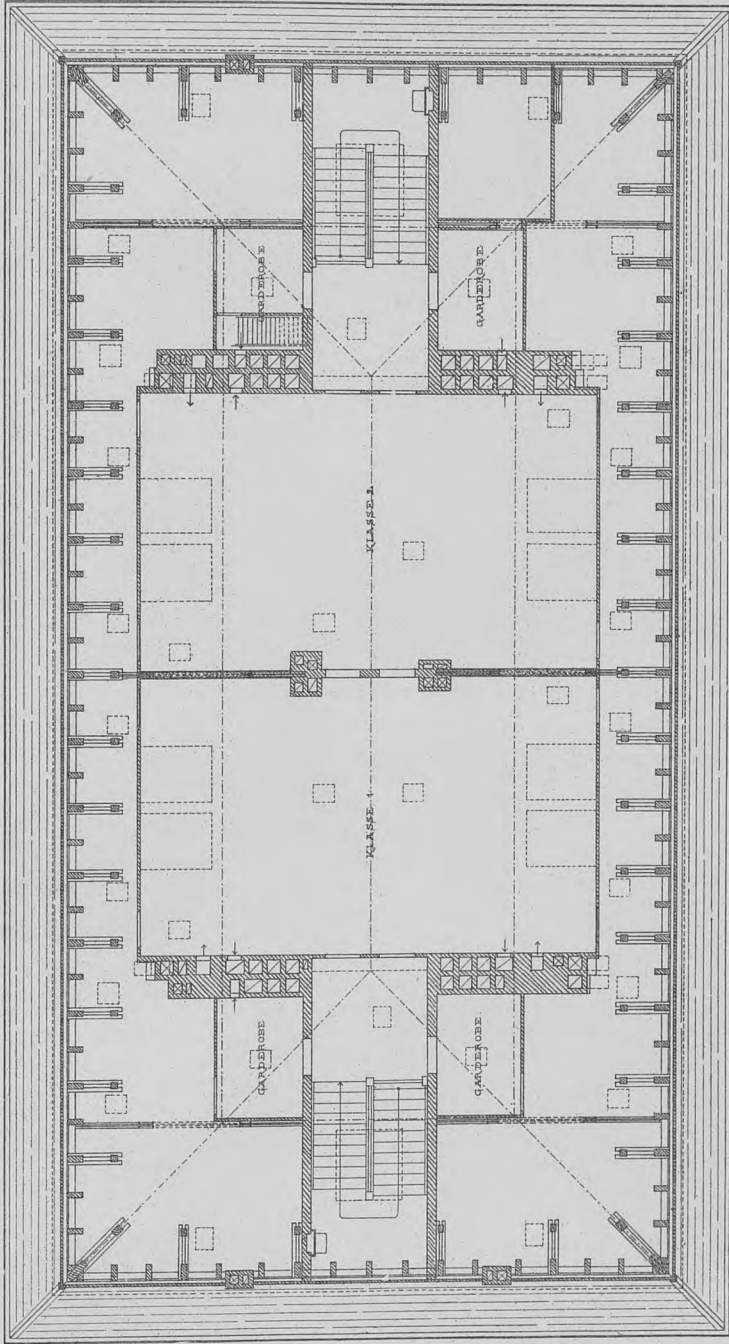
• TAGPLAN •
