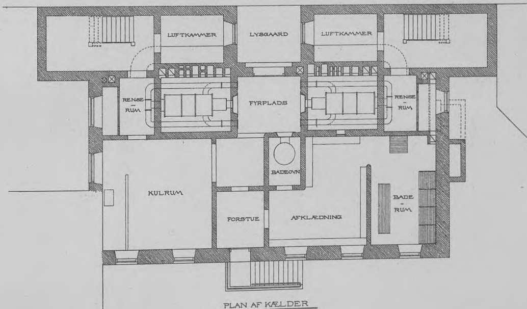
PLAN AF KÆLDER
