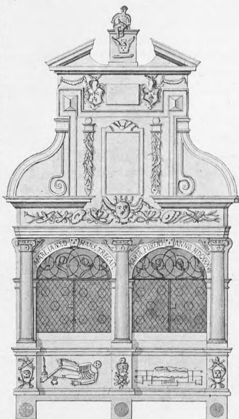
Nikolaj Kirkes Benhus. Efter Tegning i Bymuseet.
