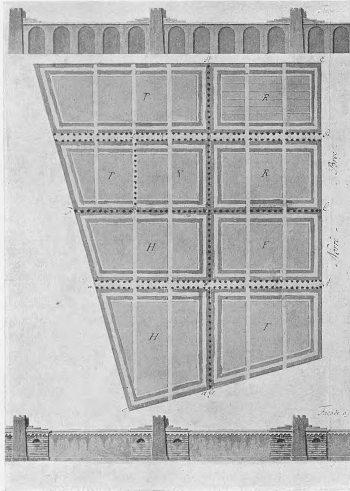
Professor Rawerts Forslag til Assistens Kirkegaards Udvidelse. Forneden Udkast til Muren ud mod Nørrebrogade, foroven samme Mur ind mod Kirkegaarden. Tegning i Raadstuearkivet.
