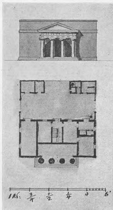
Jens Bangs Udkast til Graverboligen paa Assistens Kirkegaard. Tegning i Raadstuearkivet.
