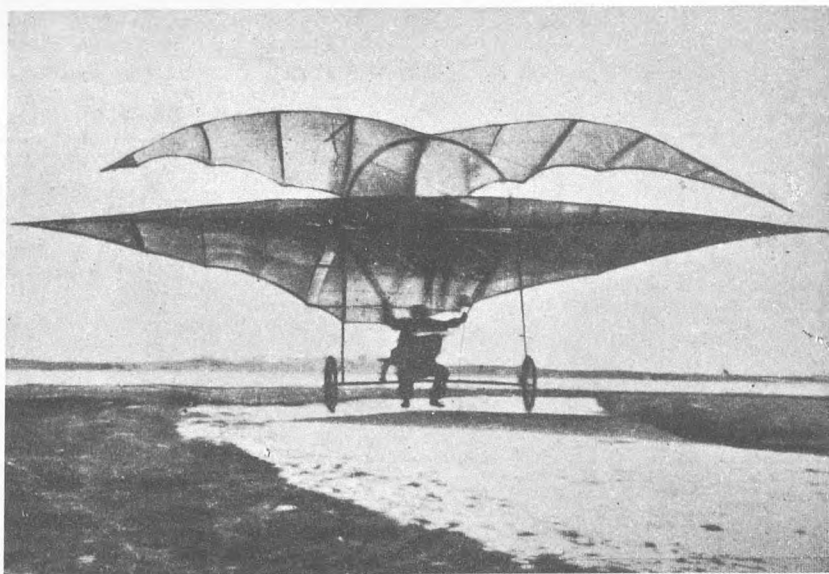
Dette er det originale Fotografi af den første Flyvning i Europa, da Ellehammer den 12. September fløj 42 Meter i 1½ Fods Højde over Cementbanen paa Lindholmen.
