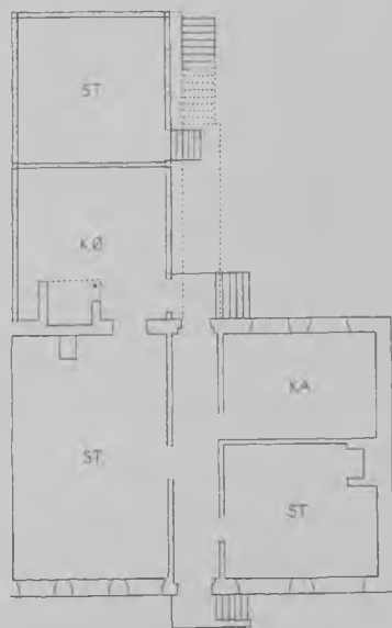
Strandgade 30 opført mellem 1624 og 1635. Rekonstruktion 1:300 af gadeside, gårdside og etageplaner. 8
