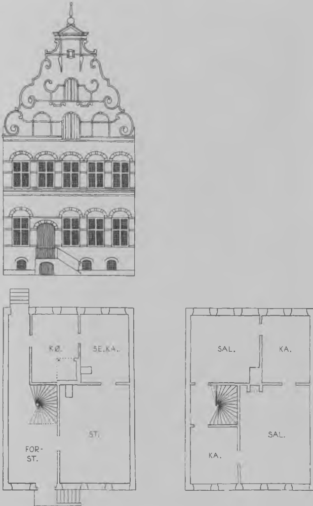
Strandgade 28 opført 1626. Rekonstruktion 1:300 bl. a. på grundlag af brandtaksation 1782.
