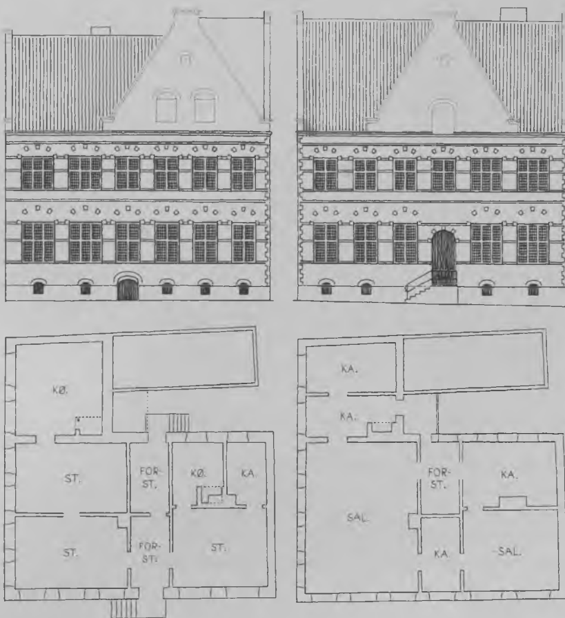
Strandgade 14 formentlig opført kort før 1650. Gadesider (Strandgade t. højre og Torvegade t. venstre) og etageplaner 1:300. Rekonstruktionsforsøg omkring 1650 for salsetagens vedkommende. Stueplanen viser indretningen i 1728 efter etableringen af de særskilte lejligheder i bygningens søndre halvdel. 14
