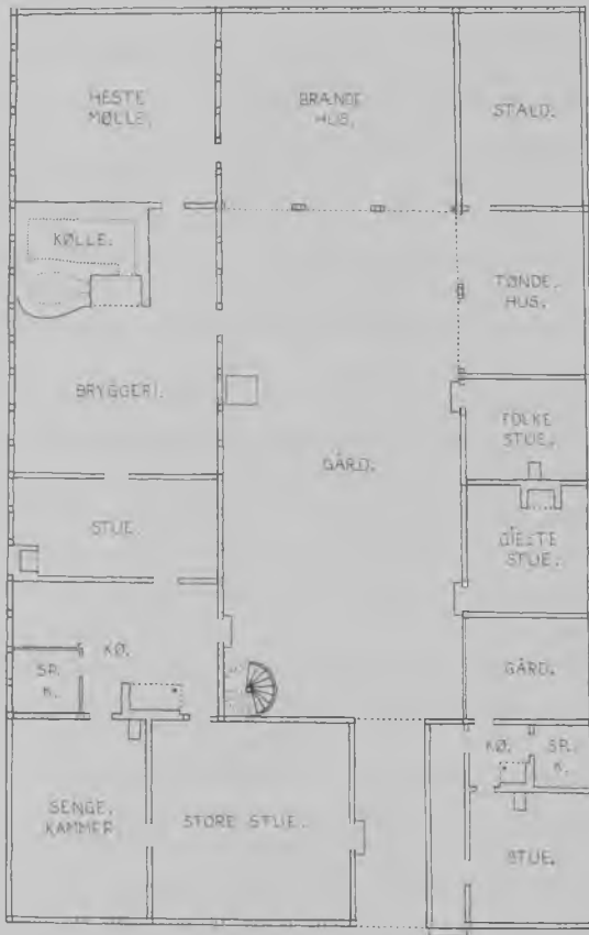
Københavnsk bryggergård. Omtegning i mål 1:300 af tømrertegning fra 1650, som viser gårdens stueplan. Originaltegningen er gengivet i H. Langberg: Tre huse på Christianshavn. Foreningen til gamle Bygningers Bevaring, årsskrift 1976.
