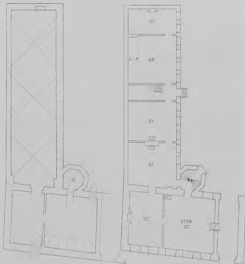
Mathias Hansens gård på Amagertorv opført 1616. Rekonstruktion af kælder- og stueplan 1:300 (vurderingsforretn. 1727). 1
