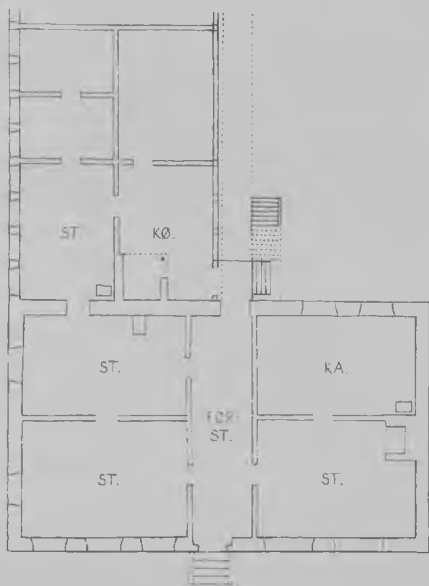
Strandgade 32 opført mellem 1624 og 1635. Rekonstruktion 1:300 af etageplaner. Efter Holger Windfeldt Schmidt. 10
