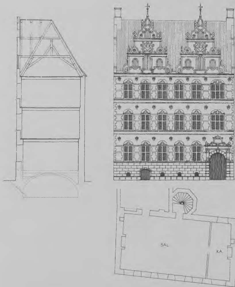
Mathias Hansens gård på Amagertorv opført 1616. Forhusets gadeside, tværsnit og salsplan. Rekonstruktion 1:300. 1
