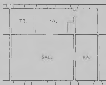
»De syv Søstre«. Spekulationsbyggeri opført mellem 1647 og 1651 af rentemester Henrik Müller. Rekonstruktion 1:300, for facadens vedkommende af et dobbelthus og for stue- og salsplanens vedkommende af et halvt dobbelthus. 44
