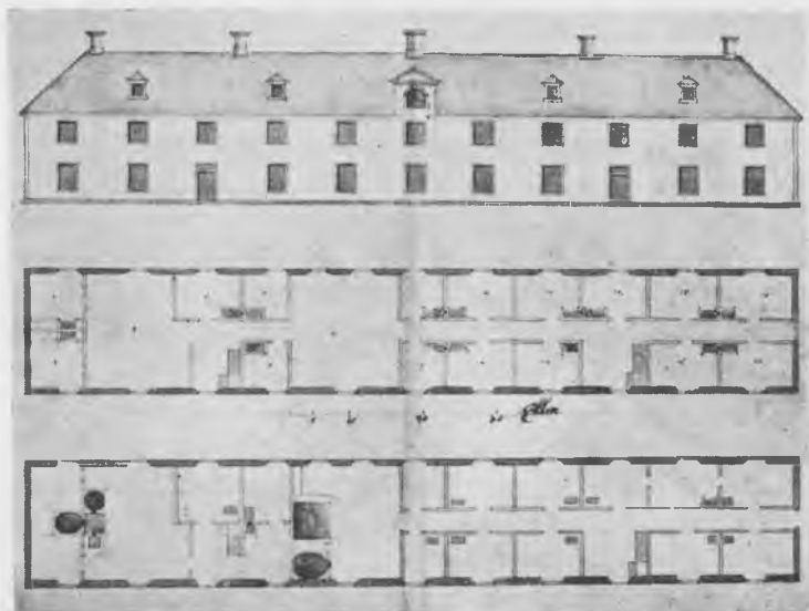
Vestfløjen på Hirschholm slot 1727. Tegningen skyldes vistnok J. C. Krieger. (Rigsark.).
