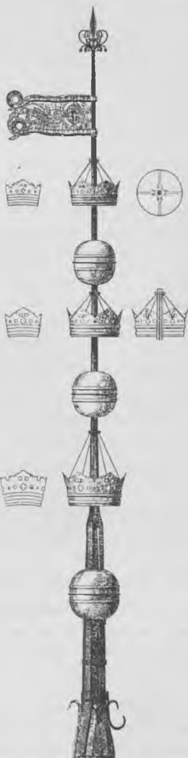
Børsspirets fløjstang. Opmåling af L. Fenger. Tidsskrift for Kunstindu- stri 1894. S. 128.
