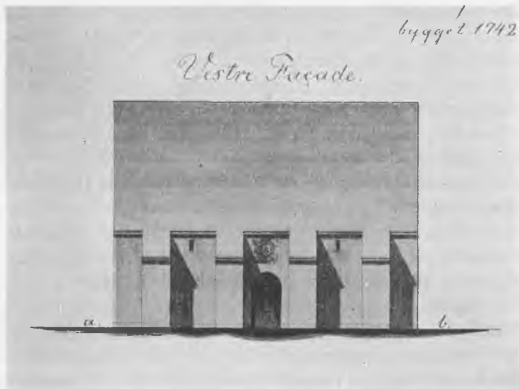
Krudttaarnet i Grevens Bastion, Kastelet. Tegning tilh. Hærens Bygningstjeneste.
