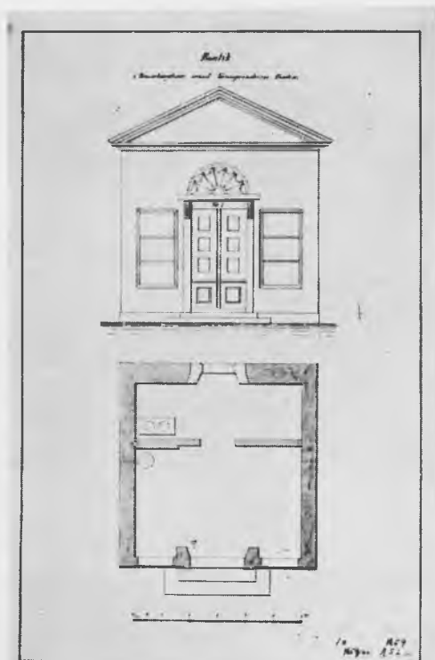
Murermester D. V. Kleins forslag fra 1859 til ombygning af pavillonerne i Kronprinsessegade.
