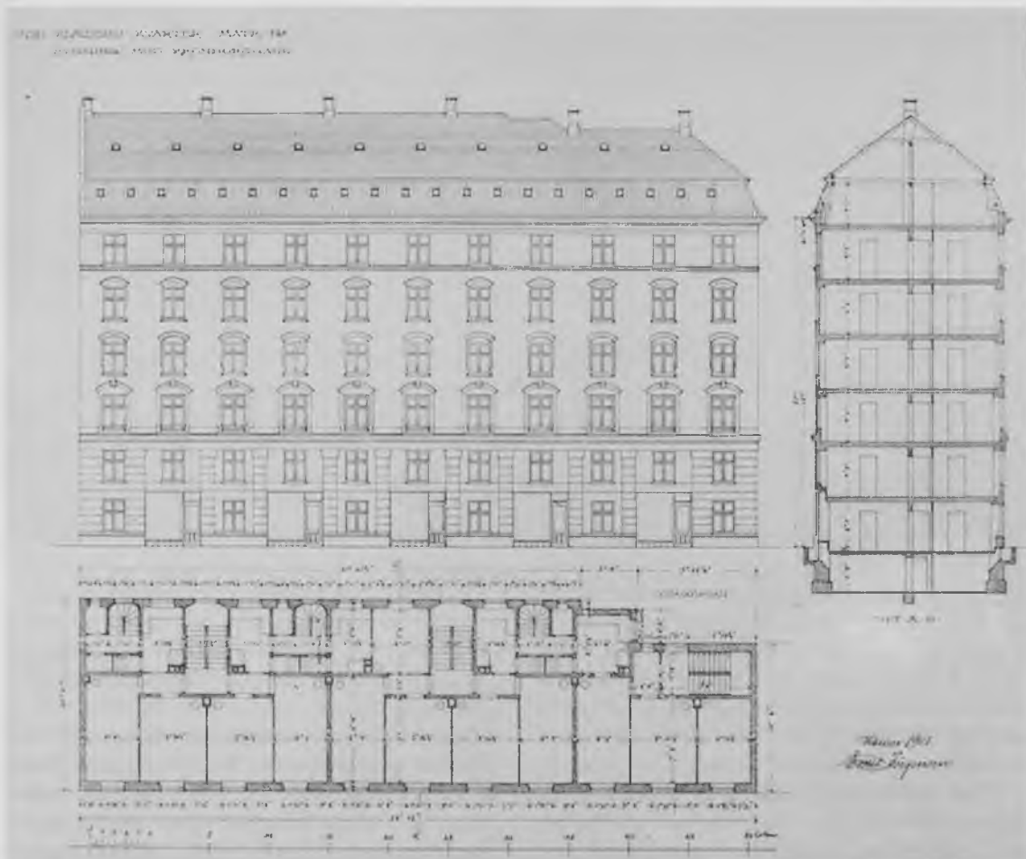
Fig. 2. Emil Jørgensen: Opstalt, plan og snit af Kronborggade 15 med de oprindelige butikker, februar 1901 (Kunstakademiets Bibliotek, Samlingen af Arkitekturtegninger).
