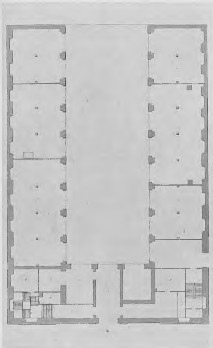
Fig. 4. Den kgl. Vogngaard, Grundplan. Da Maalestokken er udeladt, anføres her Bygningens Dimensioner. Brede 58 Alen; Længde 86 Alen; Gaardens Brede 23 Alen; Sidefløjens Brede 17\frac{1}{2} Alen.
