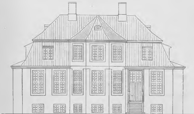
Fig. 2. Gaardfaçade. Opmaaling af Teknisk Skoles Bygnings-skole 1927—28. 1 : 200.
