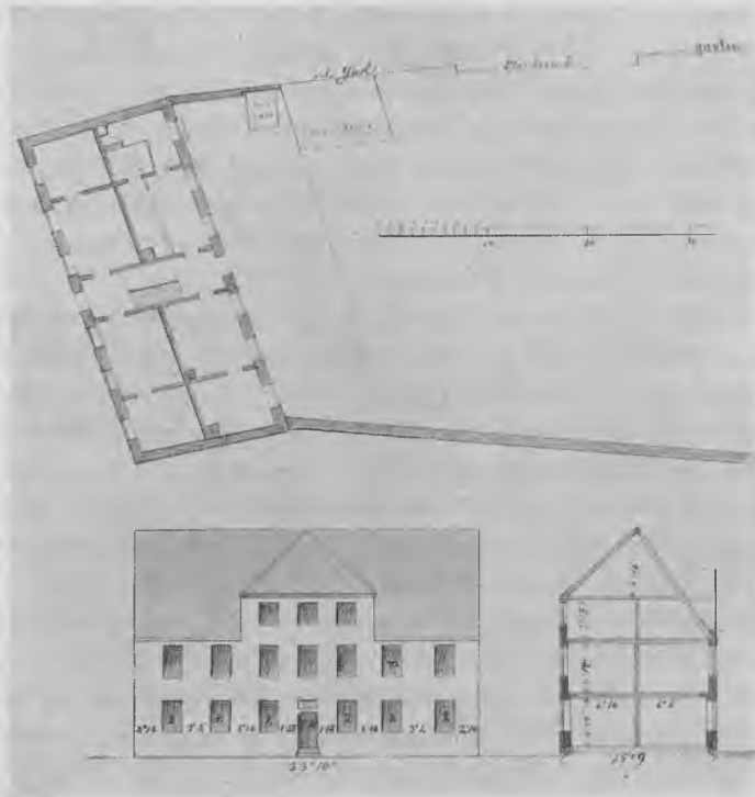
3. Opmaaling af Kollegiet før Nedrivningen i 1865. Kgl. Bibl. Kortsaml.
