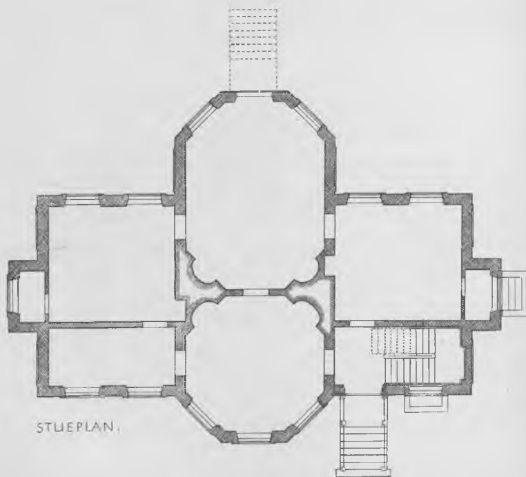
Fig. 3. Stueplan. Opmaaling af Teknisk Skoles Bygningsskole 1927—28. 1 : 200.
