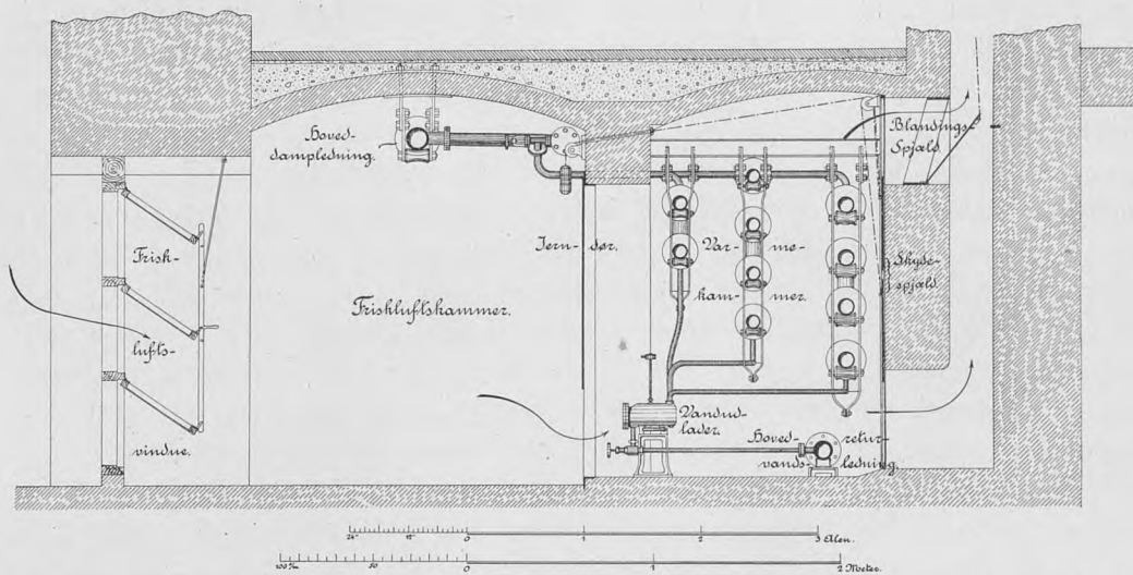
FIG. III. SKEMATISK SNIT GJENNEM ET VARMEKAMMER OG ET VARMERØR MED AUTOMATISK SPJÆLDREGULATOR
