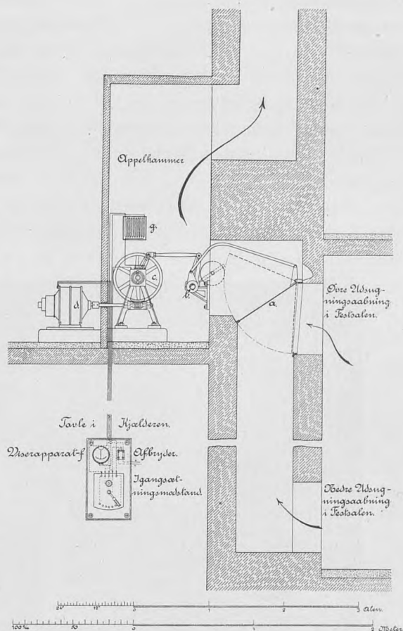
FIG. IV. SKEMATISK SNIT GJENNEM APPELUM MED FESTSALEN MED SPJÆLD OG BEVÆGMEKANISME
