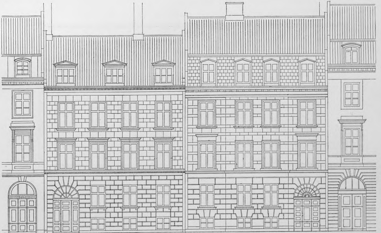
Sct. Annæ Plads Nr. 7 og Nr. 9. 1862.
