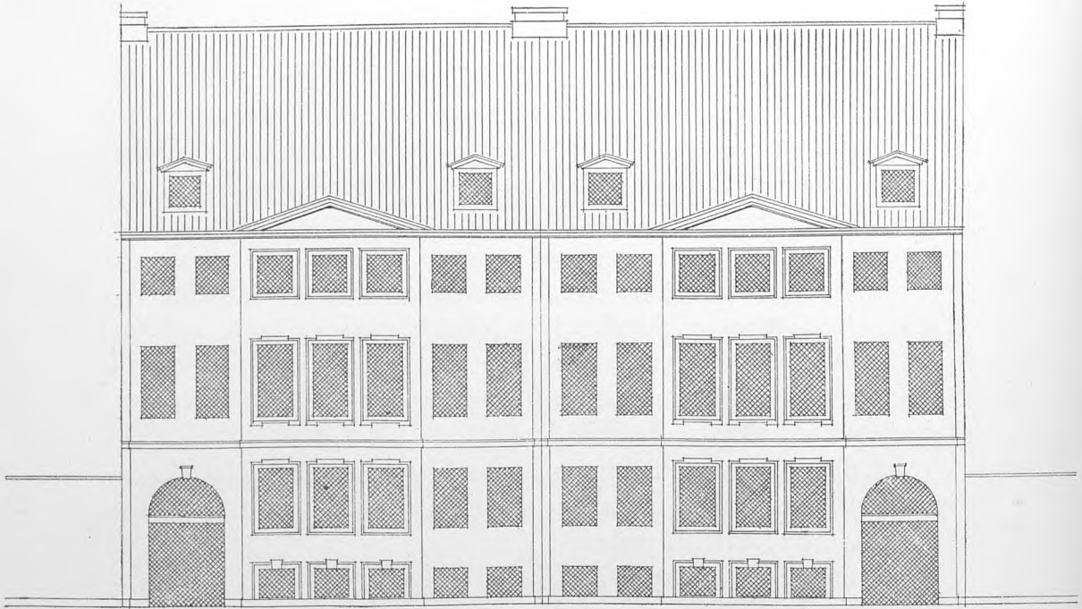
Sct. Annæ Plads Nr. 7 og Nr. 9. 1751.
