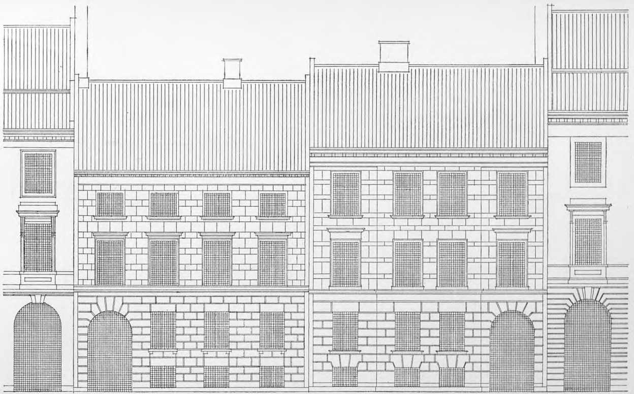
Sct. Annæ Plads Nr. 7 og Nr. 9. 1841.
