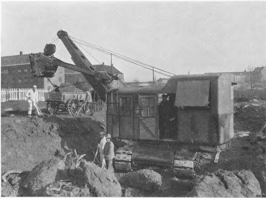
Laugets Gravemaskine i Virksomhed 1931.
