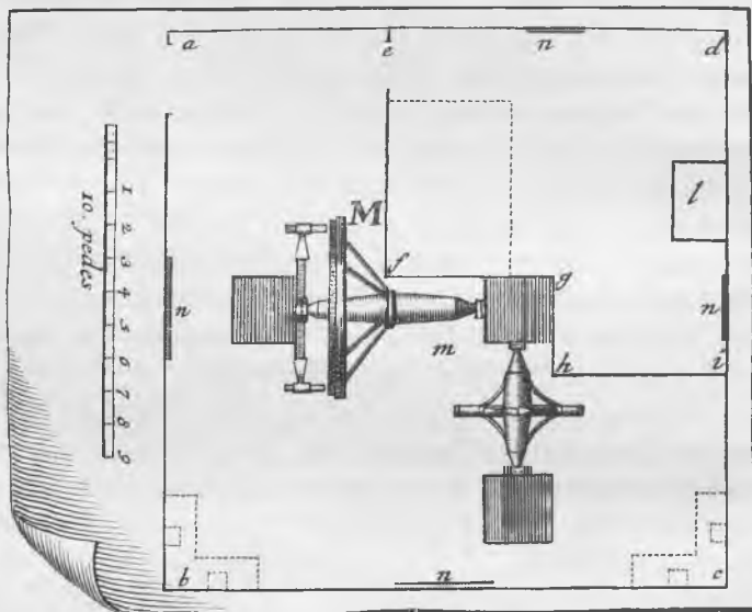
Fig. 2. Observatorium Tusculanum. c, f, g, h, i: Opholdsrum; a, e: Døre; b, c: 4 Ure; f: Hvilebænk.
