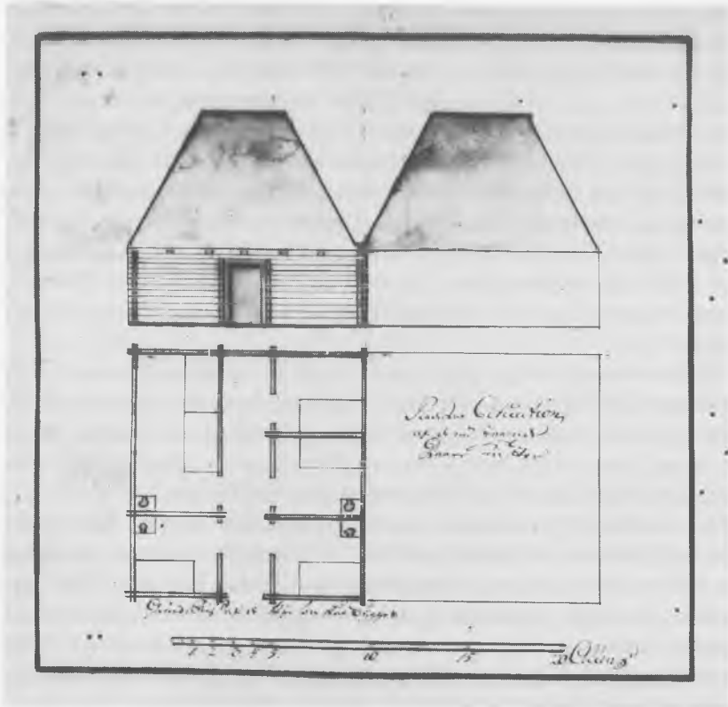
Tegning til dårekister opført ved Pesthuset. Bilag til kæmnerregnskab 1738, litra Z nr. 1, Kbh. stadsarkiv.
