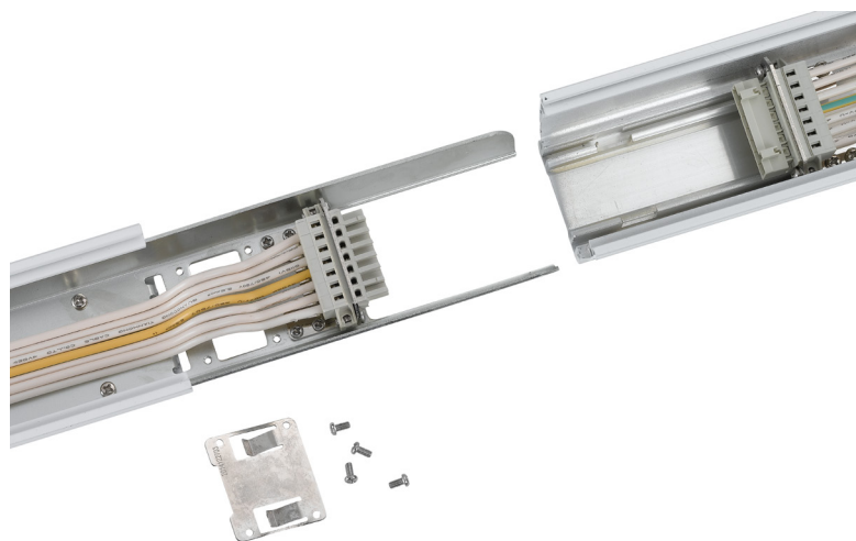
Detail Steckverbindung
