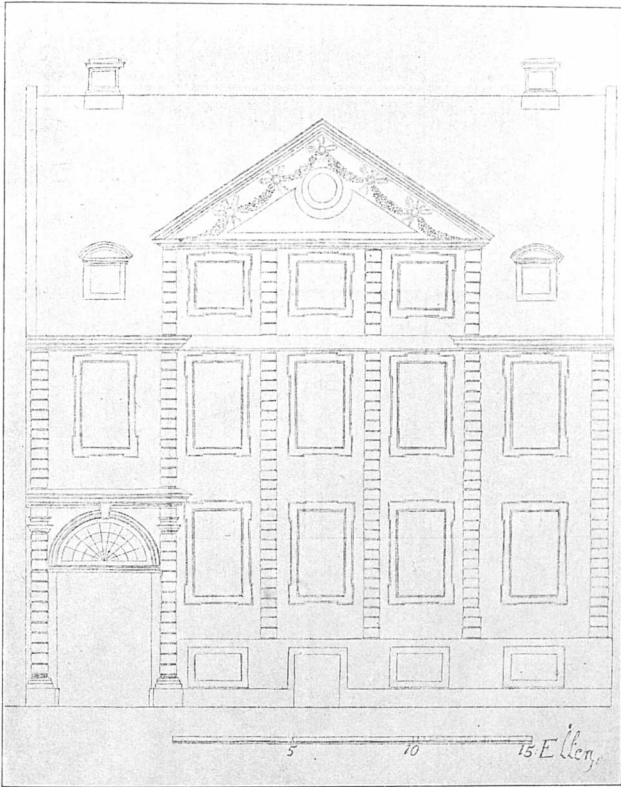
Fig. 6. Typetegning til mere anseligt Borgerhus. (Efter Krieger 1729).
