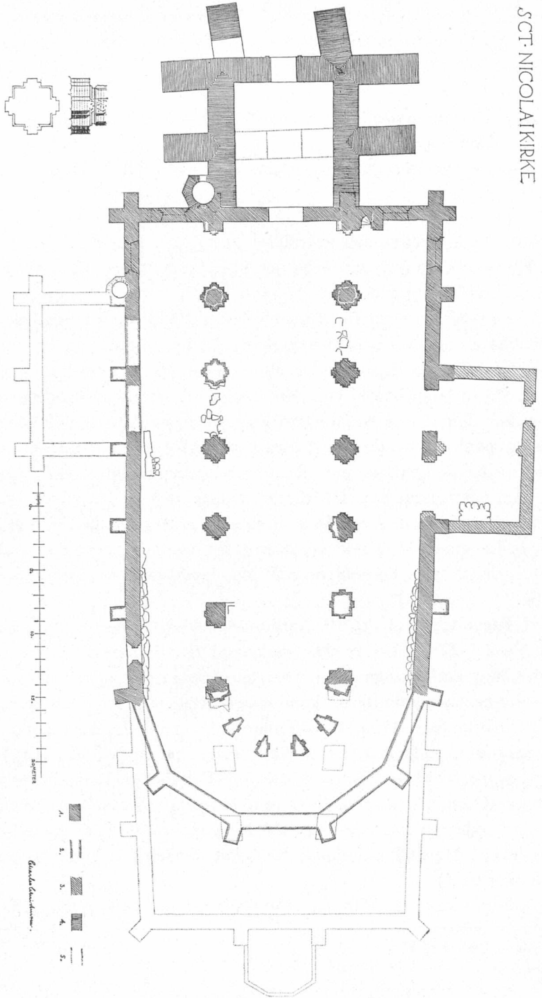
Fig. 35. Grundplan af St. Nicolaj Kirke.
