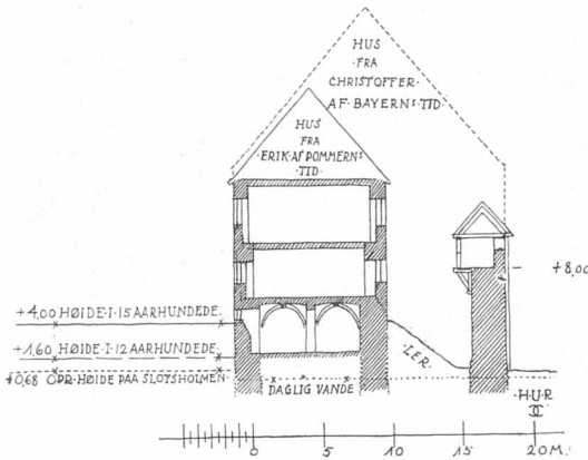
Fig. 12. Rekonstruktion af Tindemuren udfor Riddersalen.
