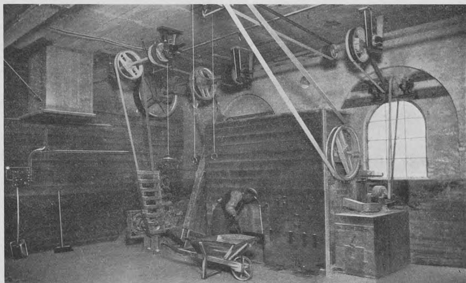
Affaldssigten
