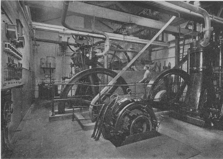
Dieselmotorer
