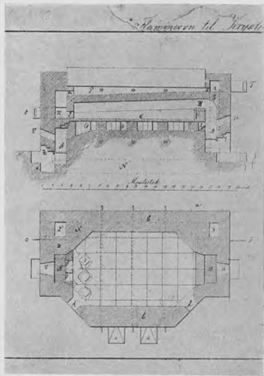
Thomsens Ovn
